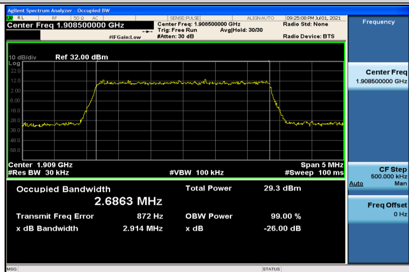
Band2-3MHz-QPSK-19185-15RB#0-2.6863
