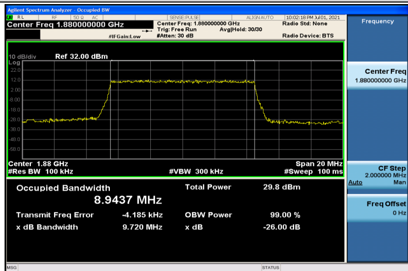
Band2-10MHz-QPSK-18900-50RB#0-8.9437
