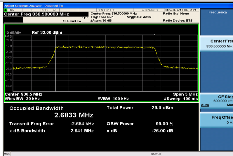
Band5-3MHz-QPSK-20525-15RB#0-2.6833
