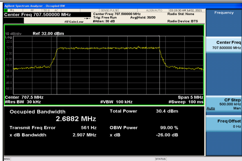
Band12-3MHz-QPSK-23095-15RB#0-2.6882
