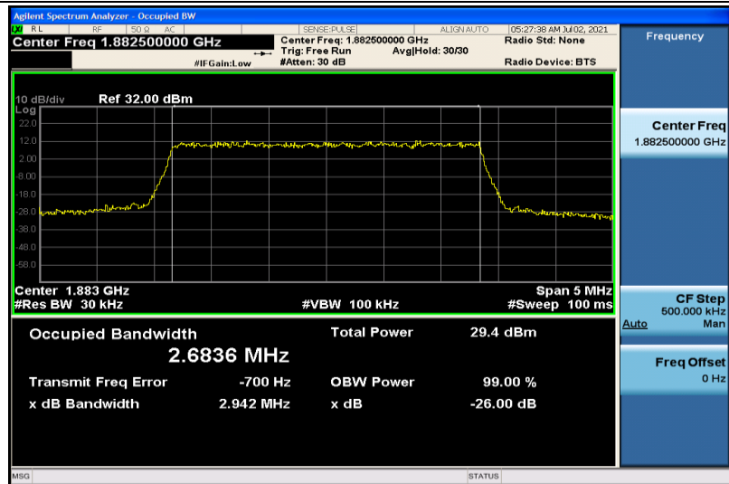
Band25-3MHz-QPSK-26365-15RB#0-2.6836
