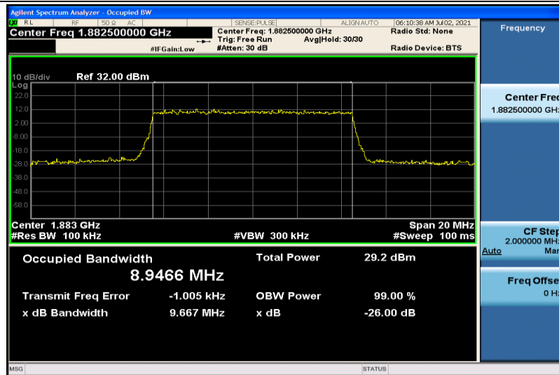
Band25-10MHz-16QAM-26365-50RB#0-8.9466
