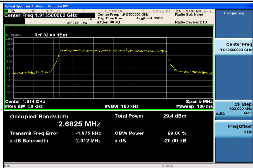
Band25-3MHz-QPSK-26675-15RB#0-2.6825
