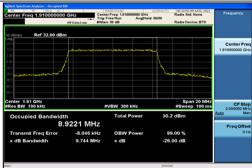
Band25-10MHz-QPSK-26640-50RB#0-8.9221
