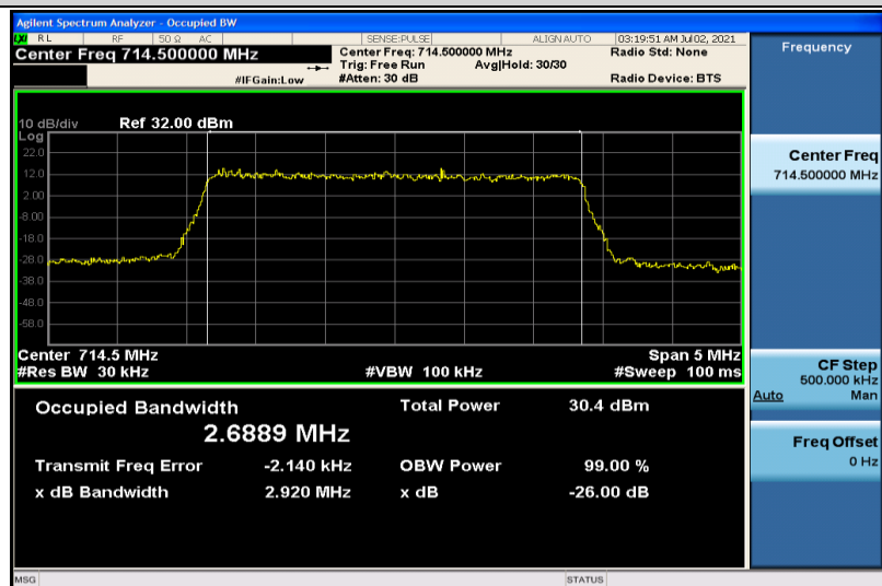
Band12-3MHz-QPSK-23165-15RB#0-2.6889
