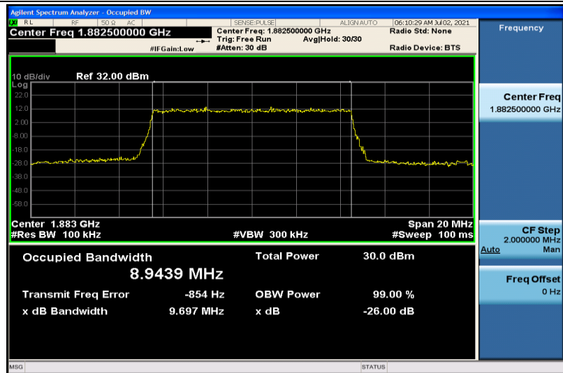
Band25-10MHz-QPSK-26365-50RB#0-8.9439
