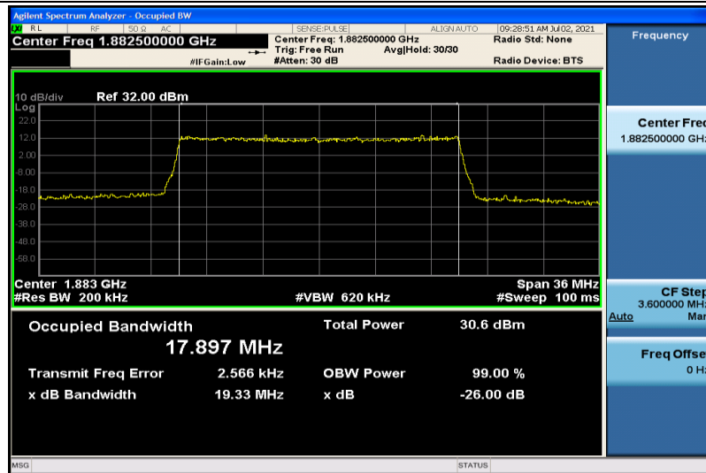
Band25-20MHz-QPSK-26365-100RB#0-17.897
