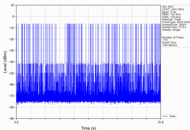
8DPSK_3DH5_HOPP_Ant1_NTNV
