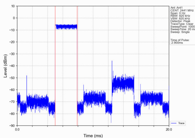
8DPSK_3DH5_HOPP_Ant1_NTNV
