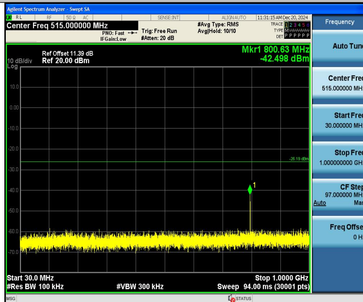
2.4G -Ant1-2402-30~1000-PASS
