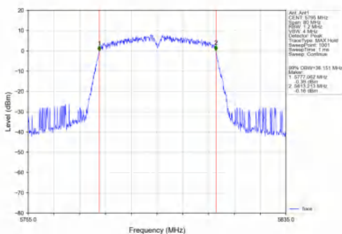
802.11n(HT40)_HCH_5795MHz_Ant1_NTNV
