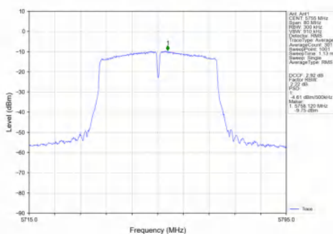
802.11ac(VHT40)_LCH_5755MHz_Ant1_NTNV
