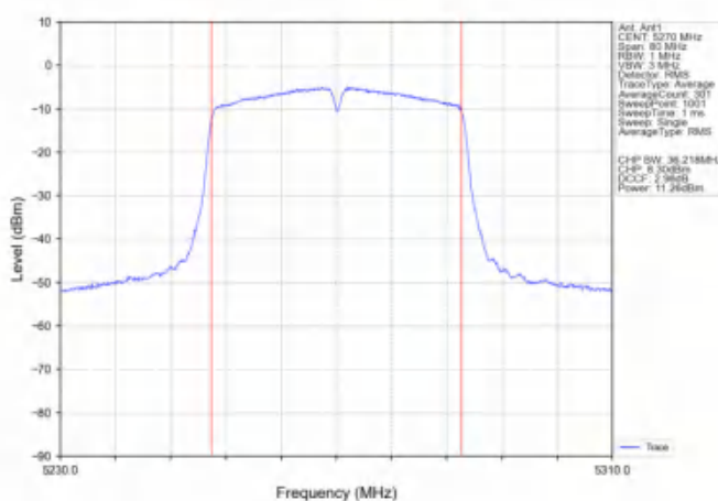
802.11n(HT40)_LCH_5270MHz_Ant1_NTNV
