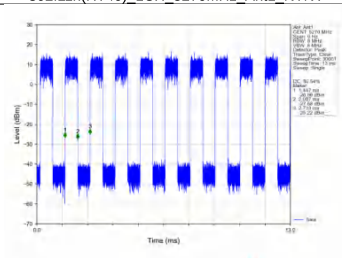
802.11n(HT40)_LCH_5270MHz_Ant1_NTNV
