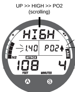
Fig. 65 - High PO2 Alarm Main
