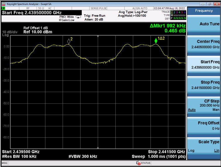
8DPSK
