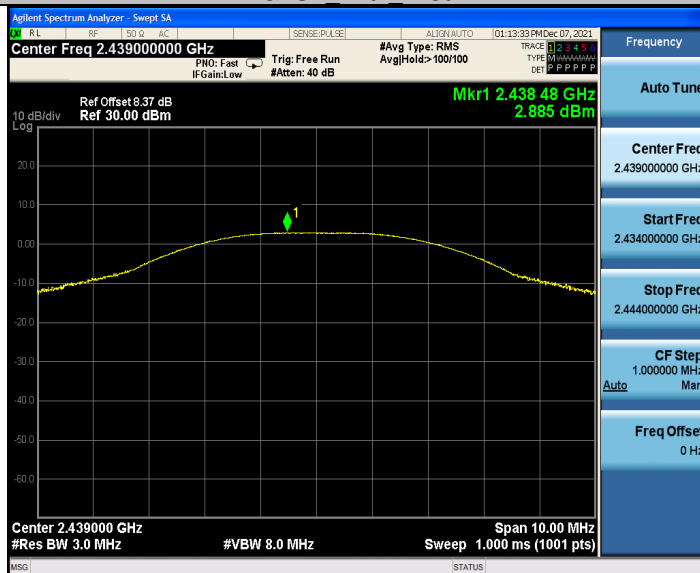
GFSK_Ant1_2439
