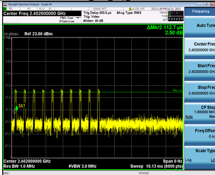
2.4G_Ant1_Hop_2402
