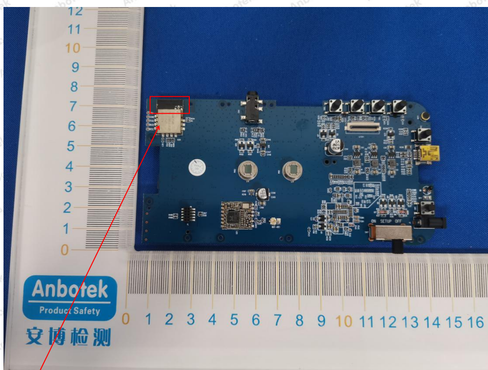
BT ANT
