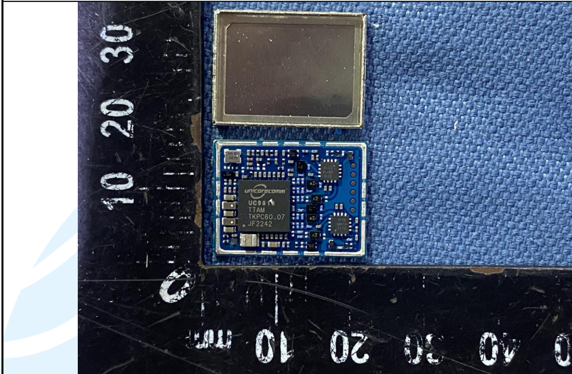
EUT Photo (GNSS RX module)
