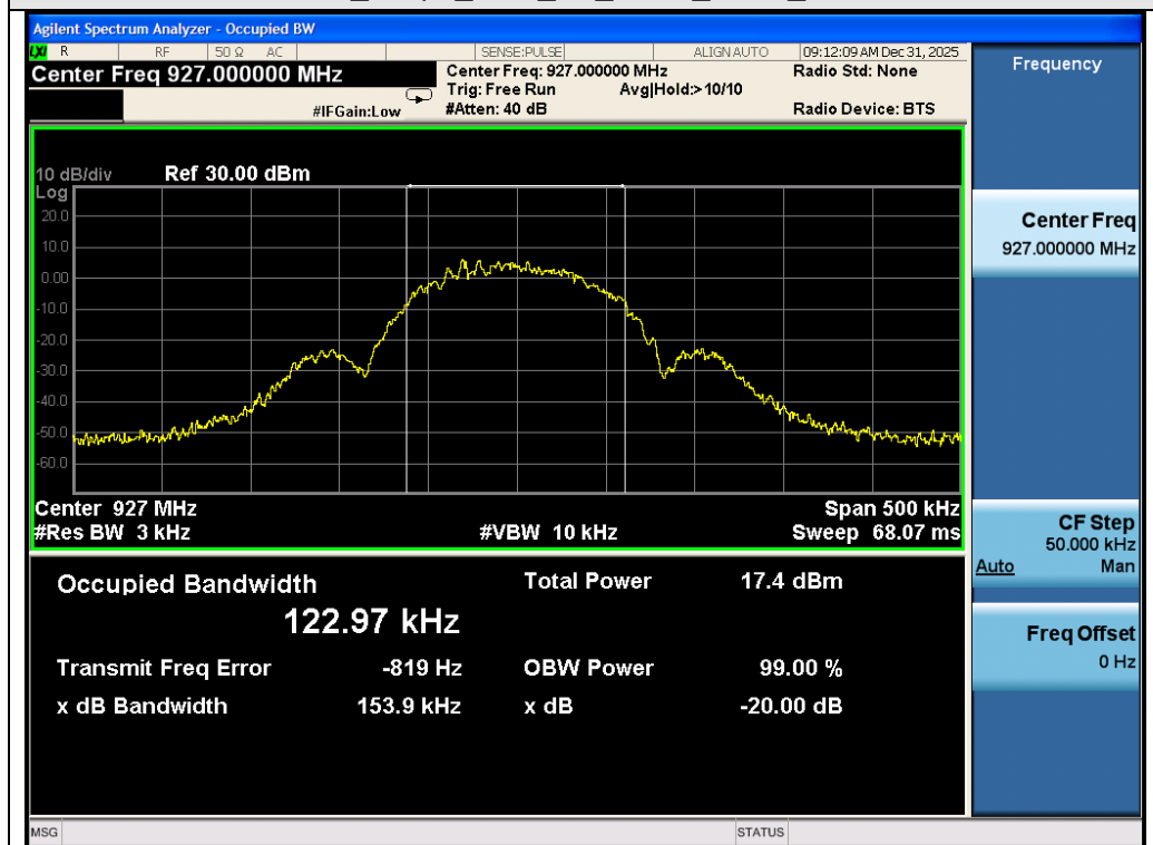
Test_Graph_SRD_TX_ANT1_927.0_OBW
