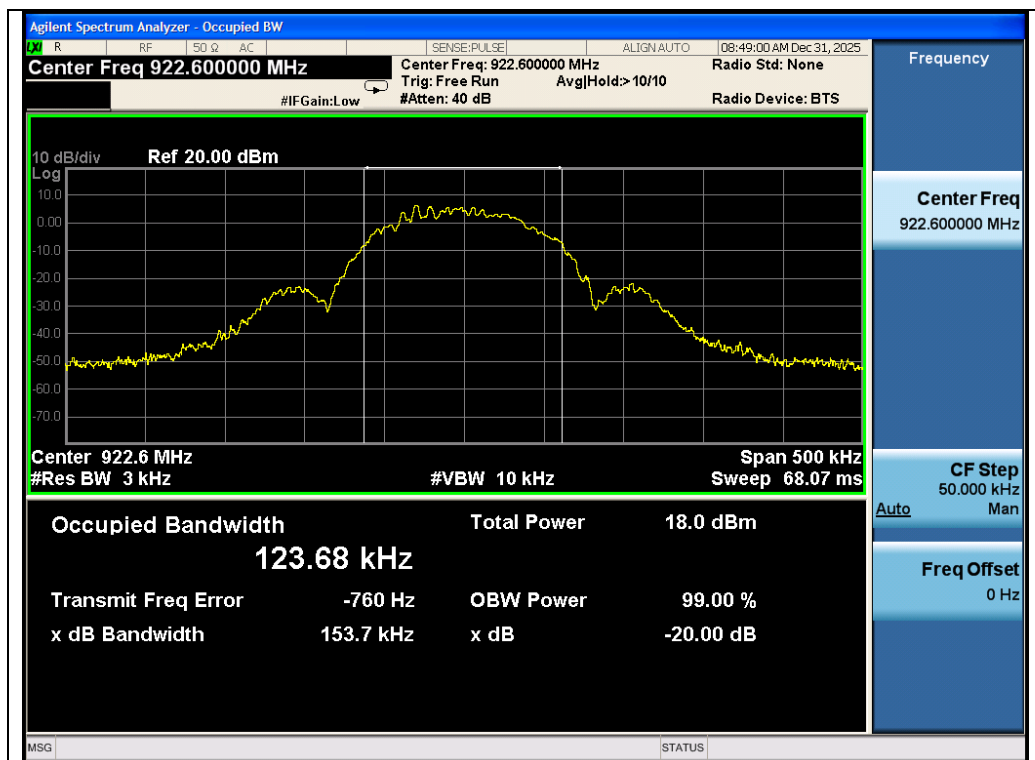
Test_Graph_SRD_TX_ANT1_922.6_OBW
