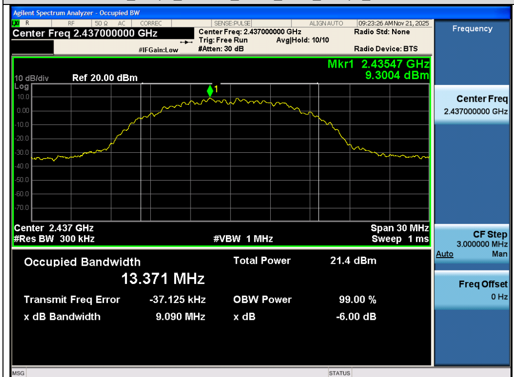
Test_Graph_802.11b_ANT1_2437_1Mbps_DTSCW
