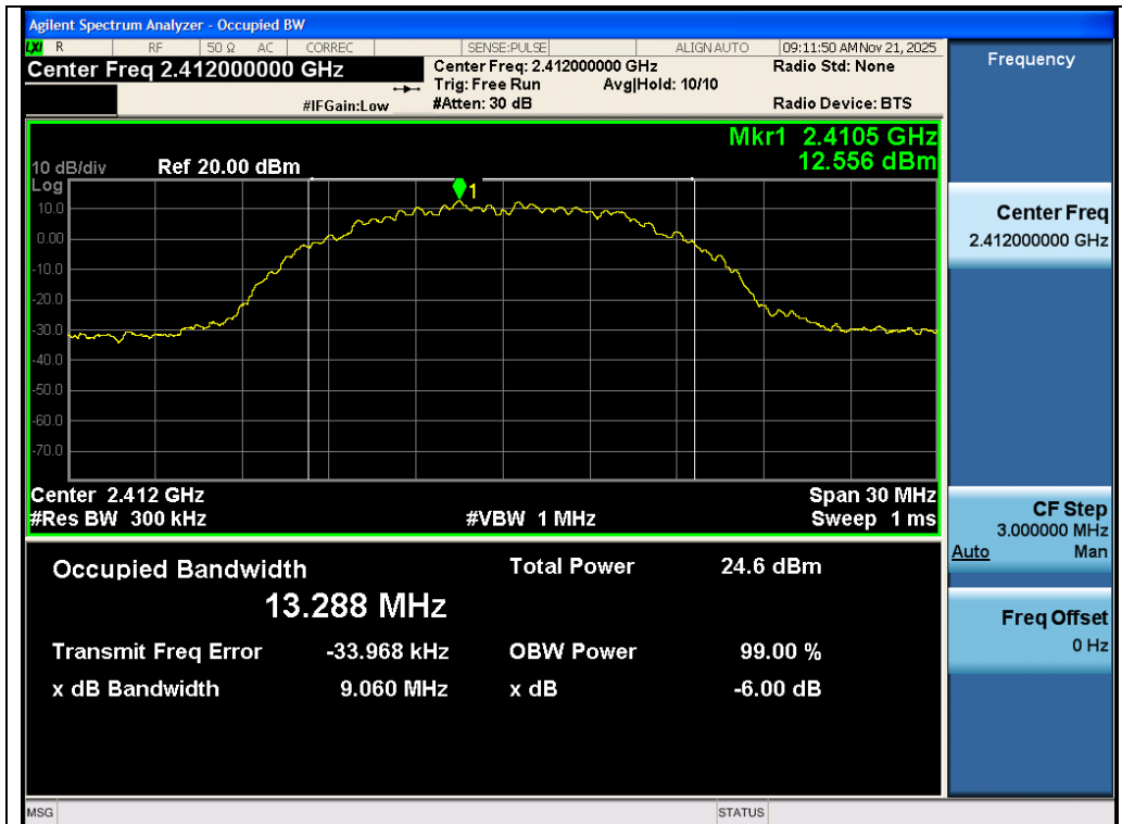
Test_Graph_802.11b_ANT1_2412_1Mbps_DTSCW
