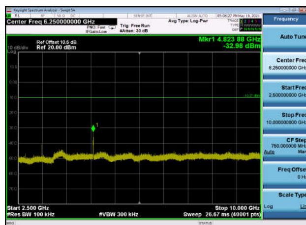
,Plot 4,2500MHz~10000MHz-802.11b ,2462MHz
