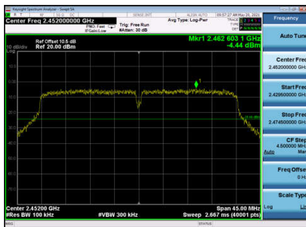
,Plot 1,Reference Level-802.11n(HT40) ,2452MHz
