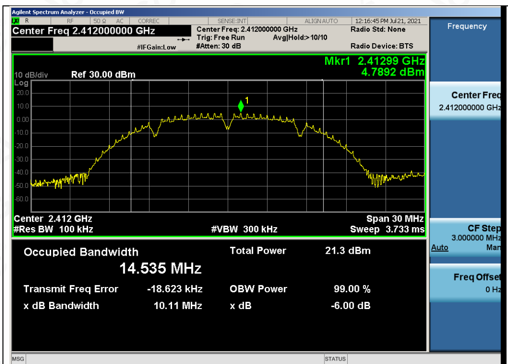
Test_Graph_802.11b_ANT2_2412_1Mbps_DTSBW
