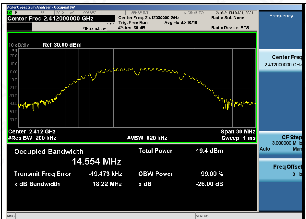
Test_Graph_802.11b_ANT2_2412_1Mbps_OBW
