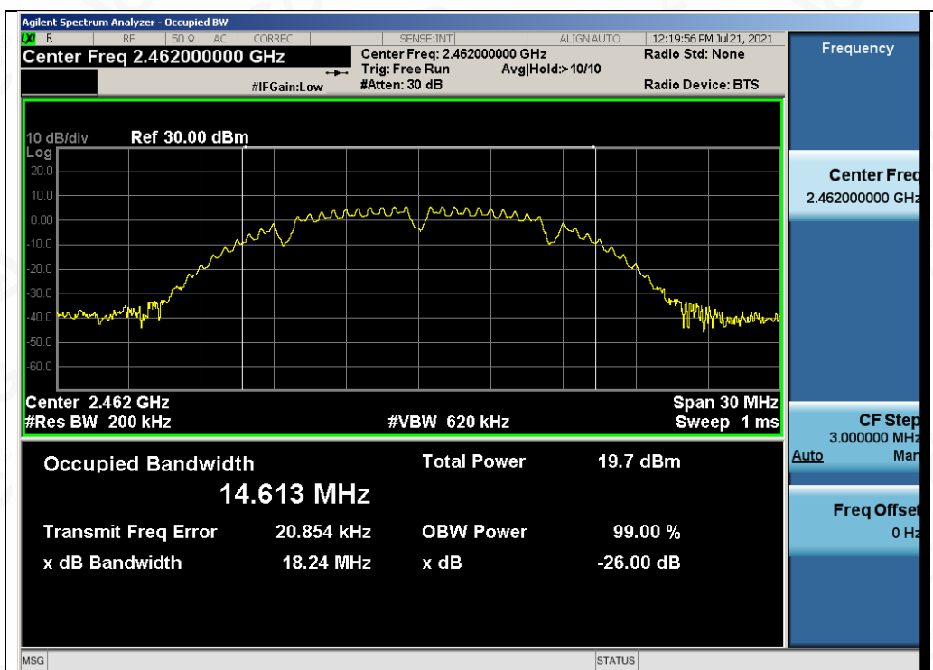
Test_Graph_802.11b_ANT2_2462_1Mbps_OBW
