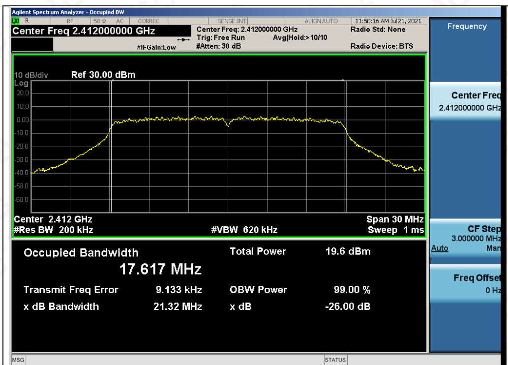
Test_Graph_802.11n20_ANT1_2412_MCS0_OBW
