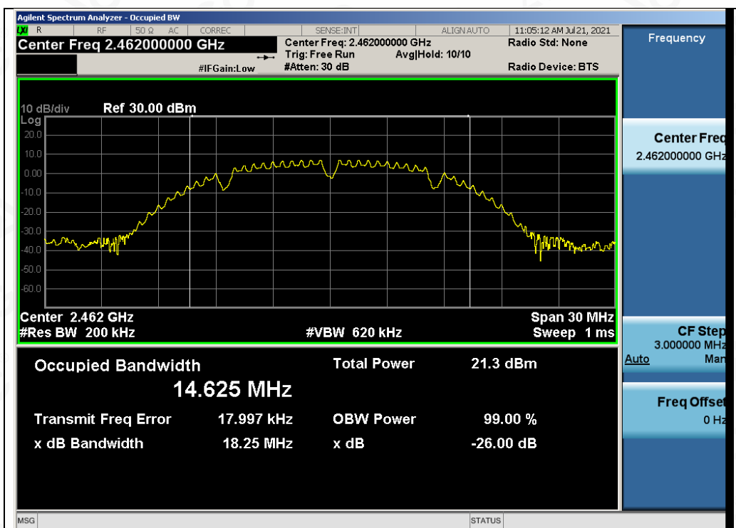
Test_Graph_802.11b_ANT1_2462_1Mbps_OBW
