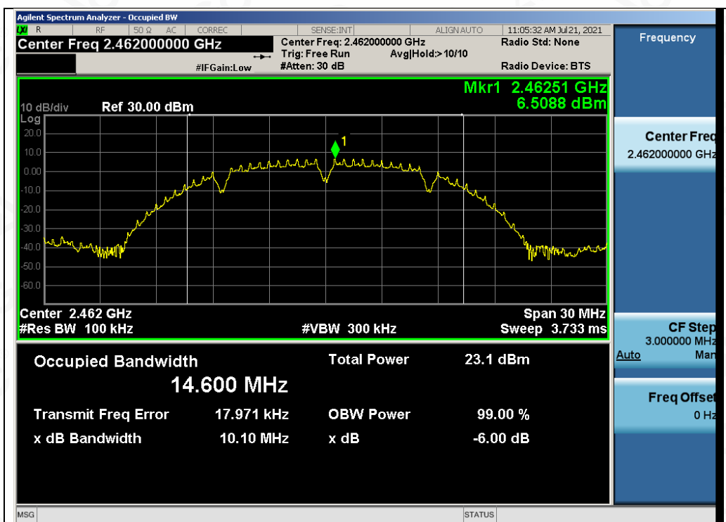
Test_Graph_802.11b_ANT1_2462_1Mbps_DTSBW
