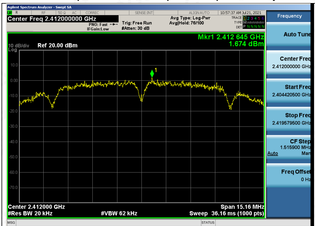
Test_Graph_802.11b_ANT1_2412_1Mbps_PSD
