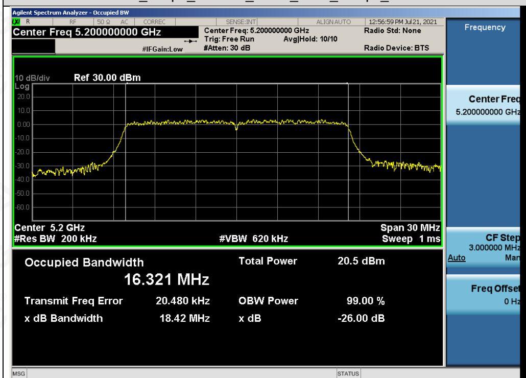
Test_Graph_802.11a_ANT1_5200_6Mbps_OBW
