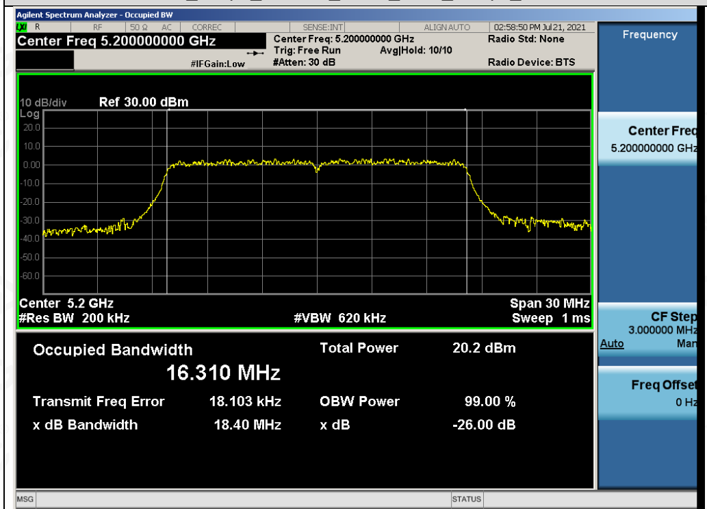
Test_Graph_802.11a_ANT2_5200_6Mbps_OBW
