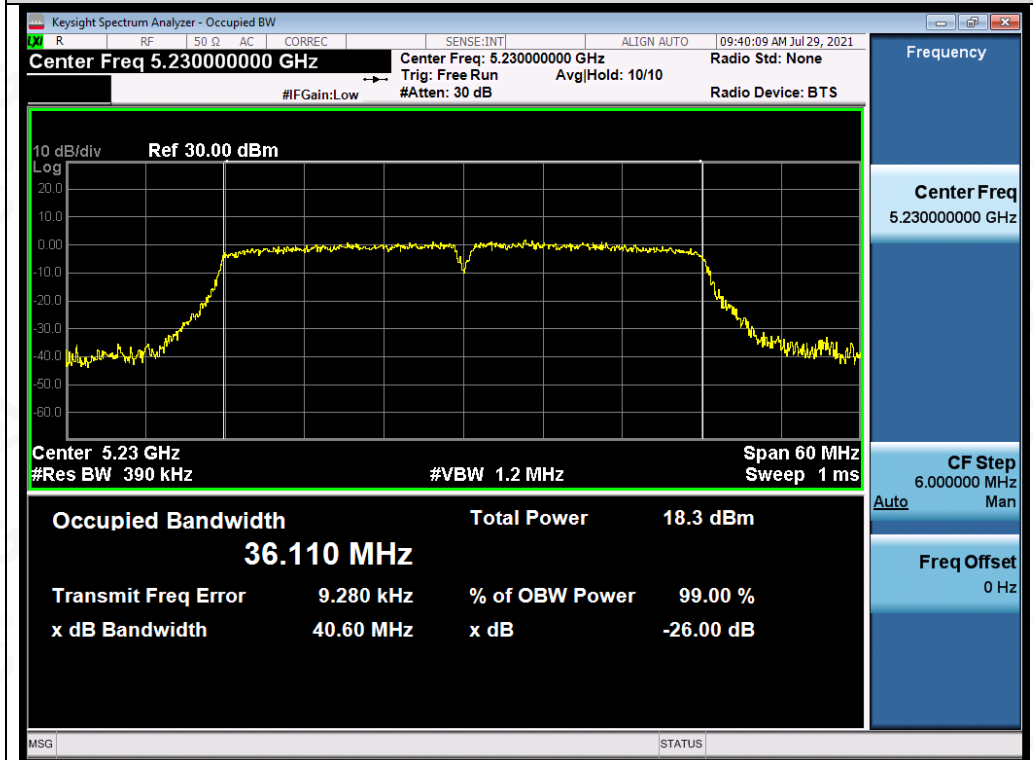
Test_Graph_802.11n40_ANT1_5230_MCS0_OBW
