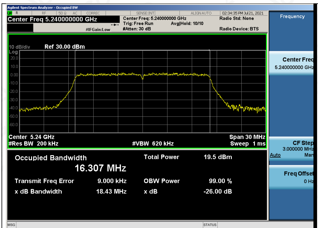
Test_Graph_802.11a_ANT1_5240_6Mbps_OBW
