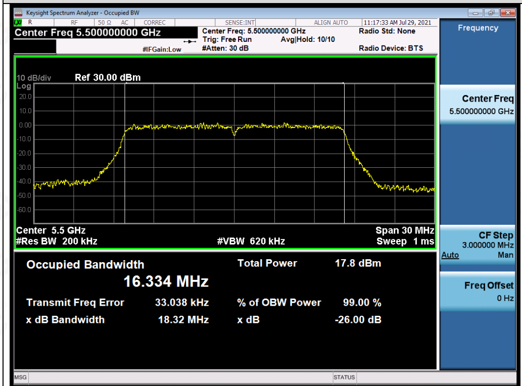
Test_Graph_802.11a_ANT2_5500_6Mbps_OBW
