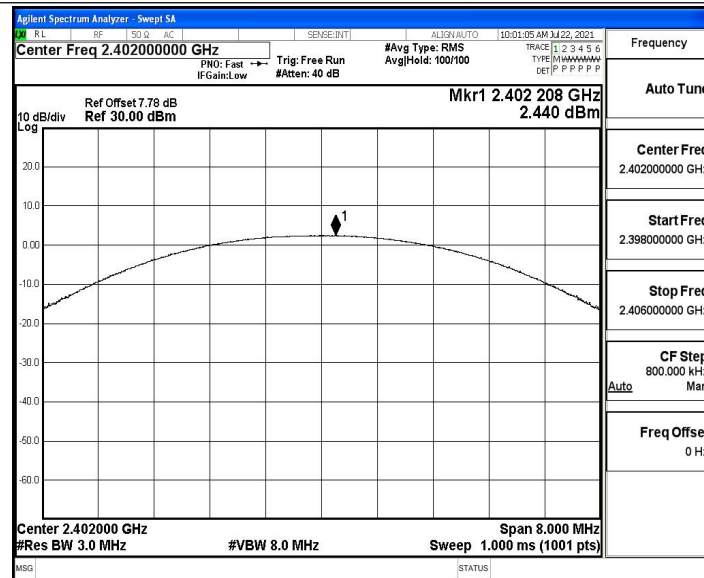
DH5_Ant1_2402
