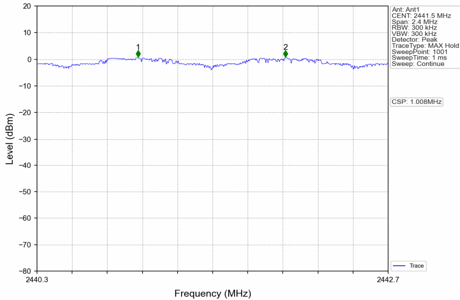
Pi/4DQPSK_2DH5_HOPP_Ant1_NTNV
