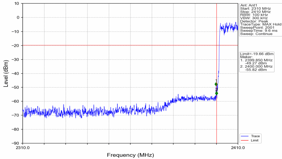
Pi/4DQPSK_2DH5_HOPP_Ant1_NTNV
