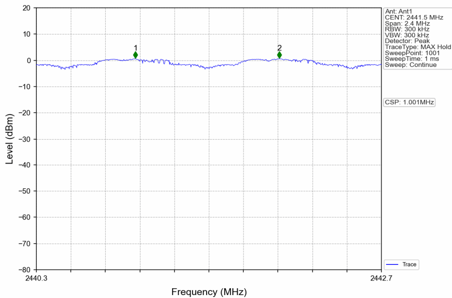
8DPSK_3DH5_HOPP_Ant1_NTNV
