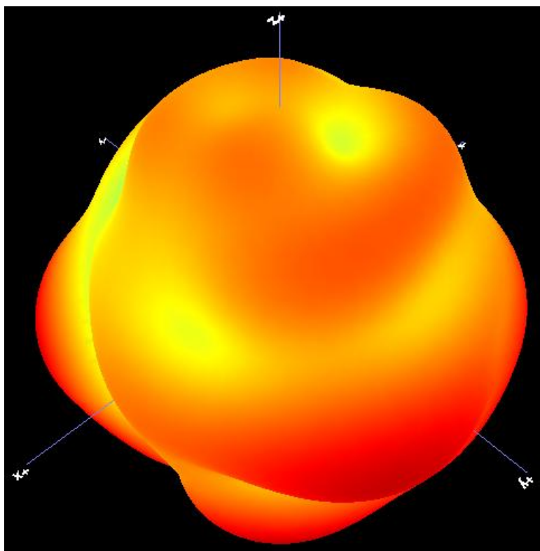
2440MHz
