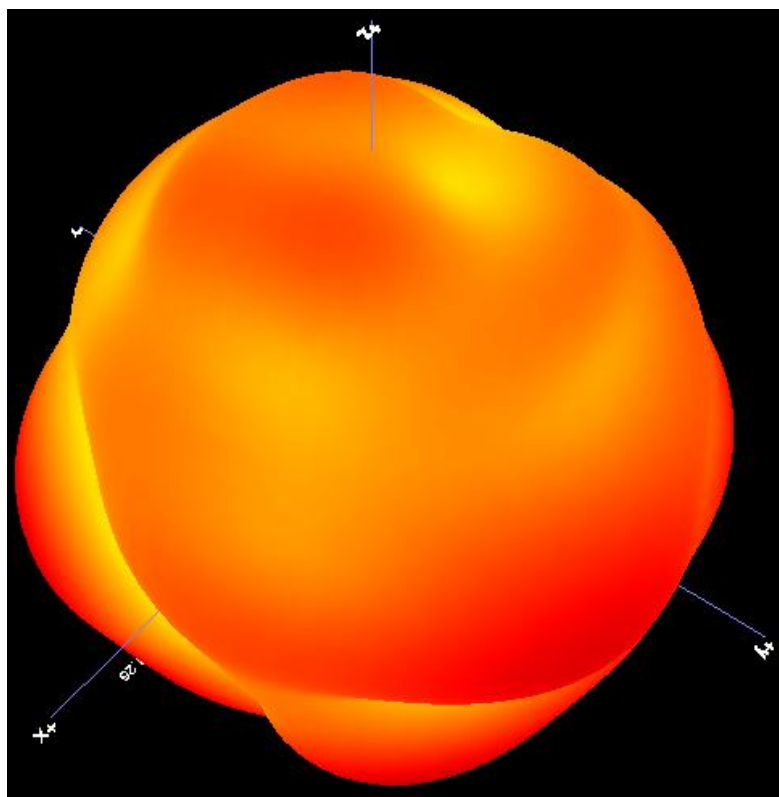
2402MHz
