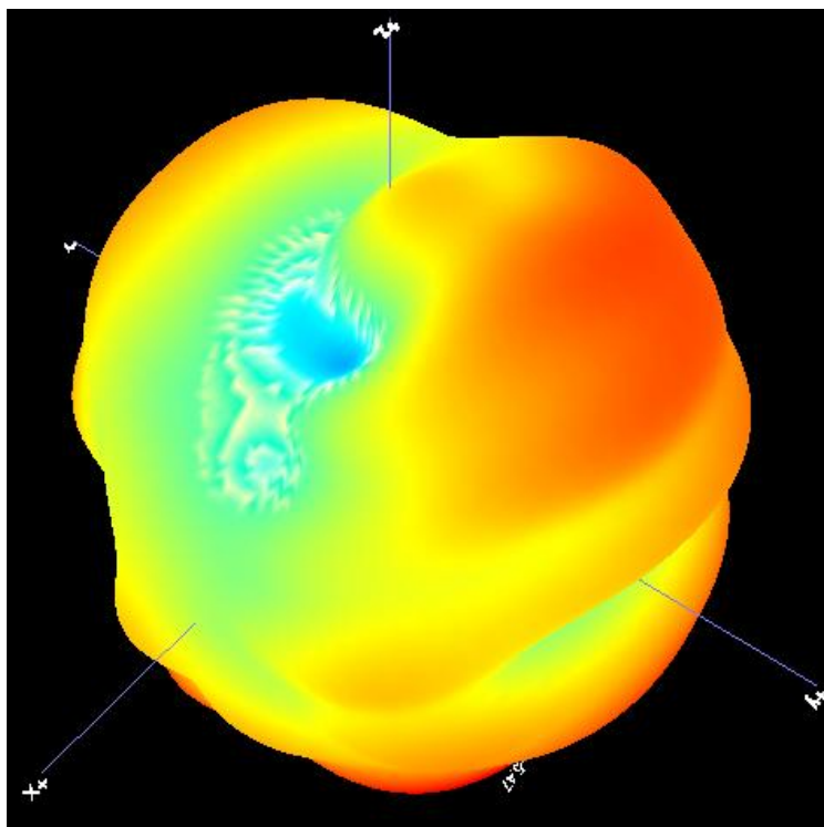
2440MHz
