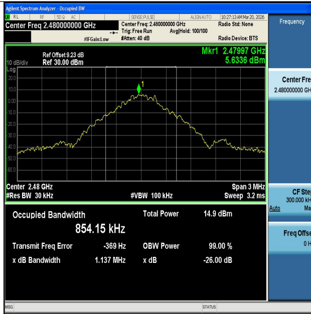
DH5-Ant1-2480
