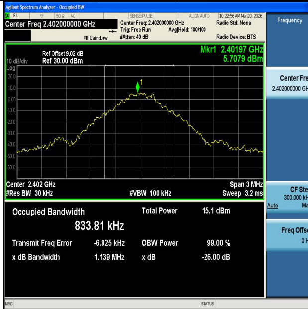
DH5-Ant1-2402
