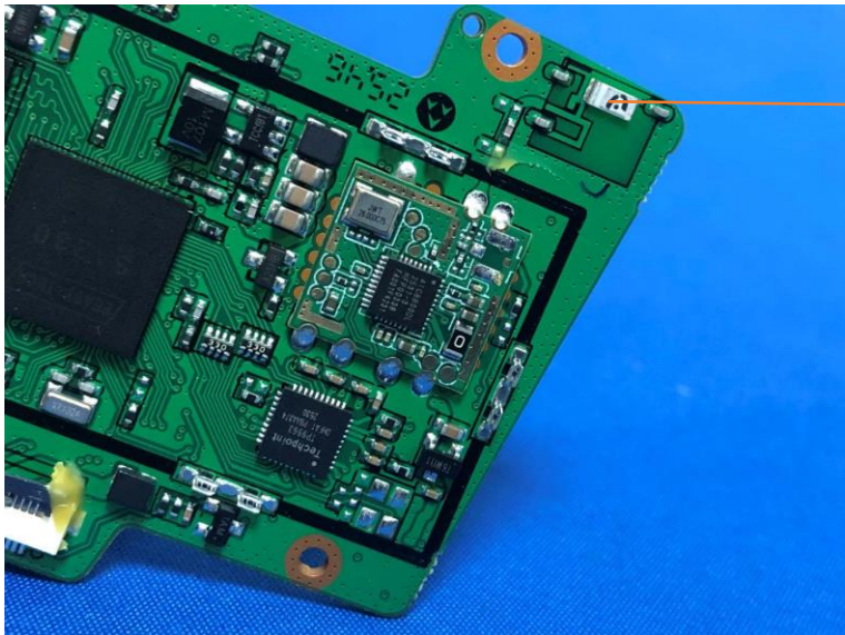
2.4GWIFI ANT
