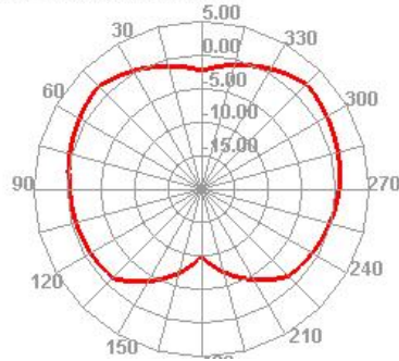
2500.000MHz H
