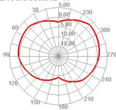
2400.000MHz H
