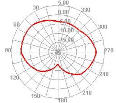
2500.000MHz E2
