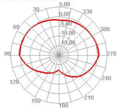
2400.000MHz E2
