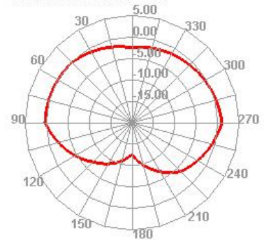
2450.000MHz E2
