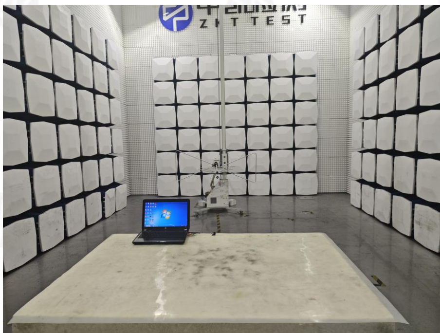
RE (1GHz-18GHz)
