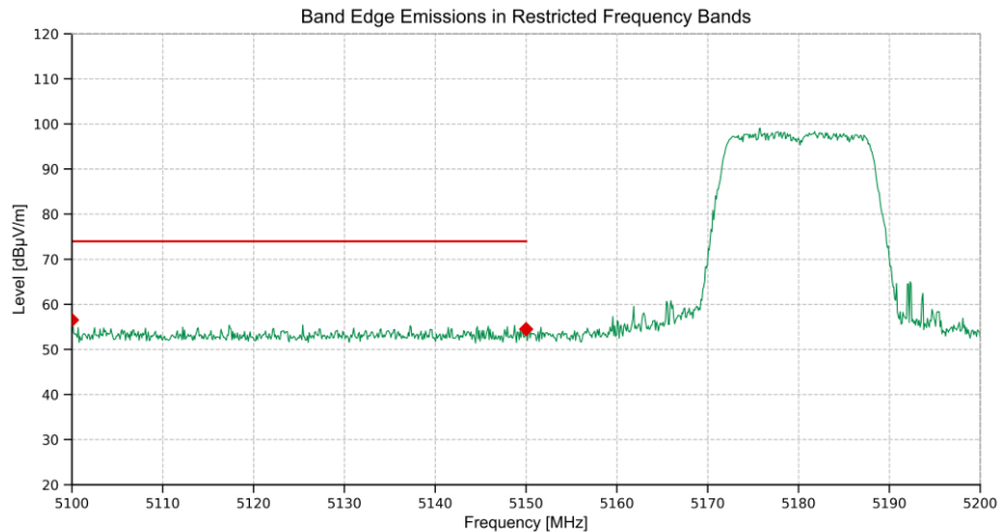
11a_ANT1_5180_6Mbps
