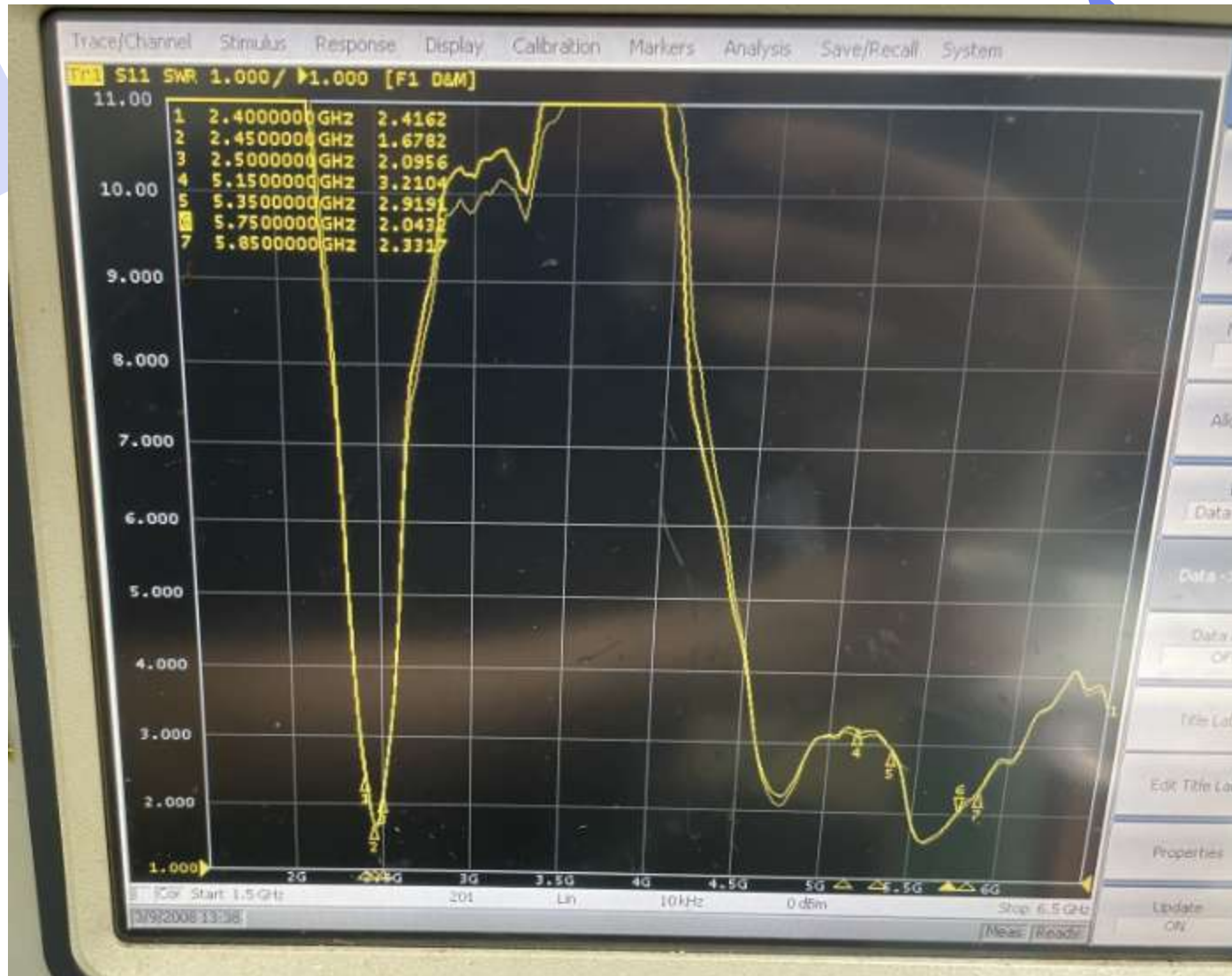
天线S11
