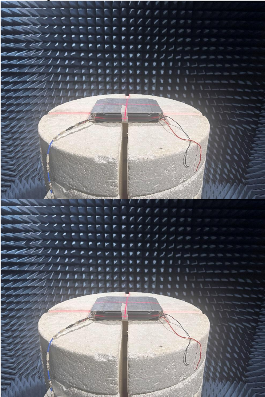
DUT Setup Photo
