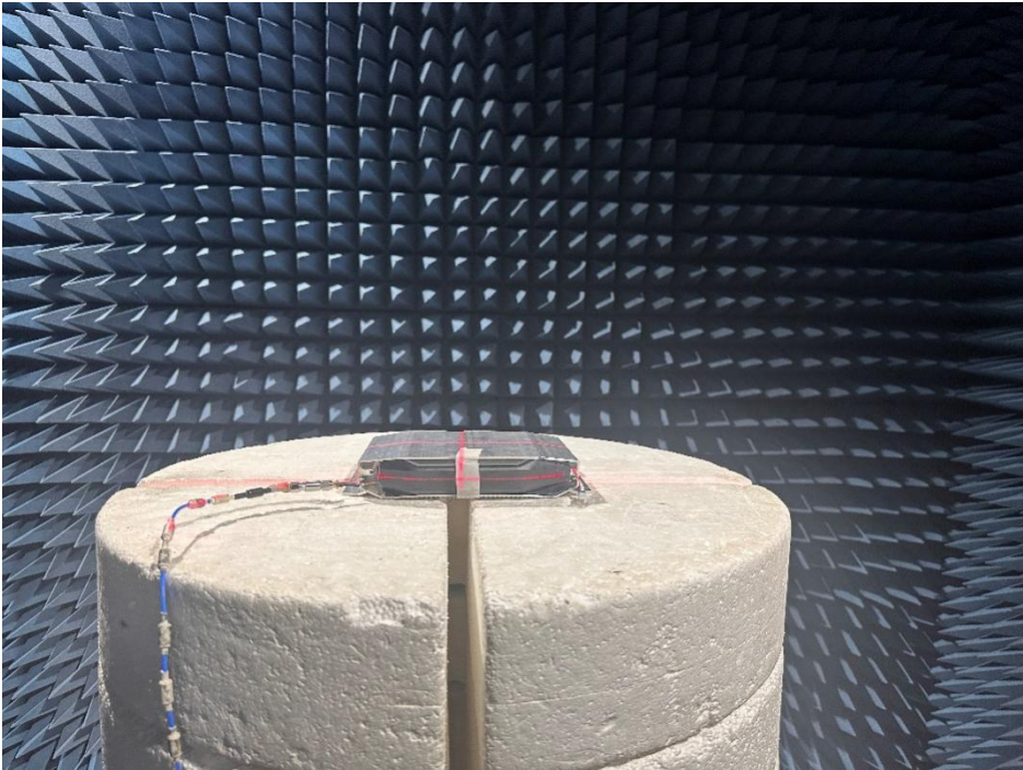
DUT Setup Photo
