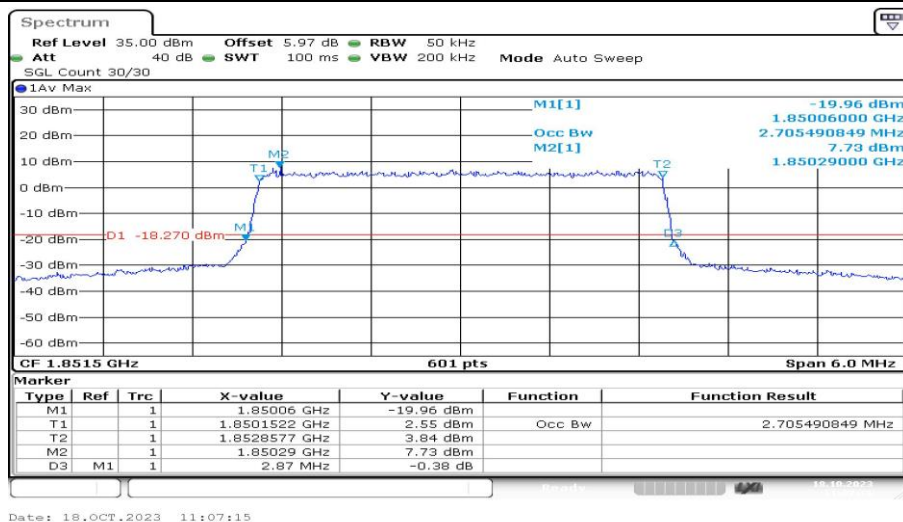
Band2-3MHz-QPSK-18615-15RB#0-PASS
