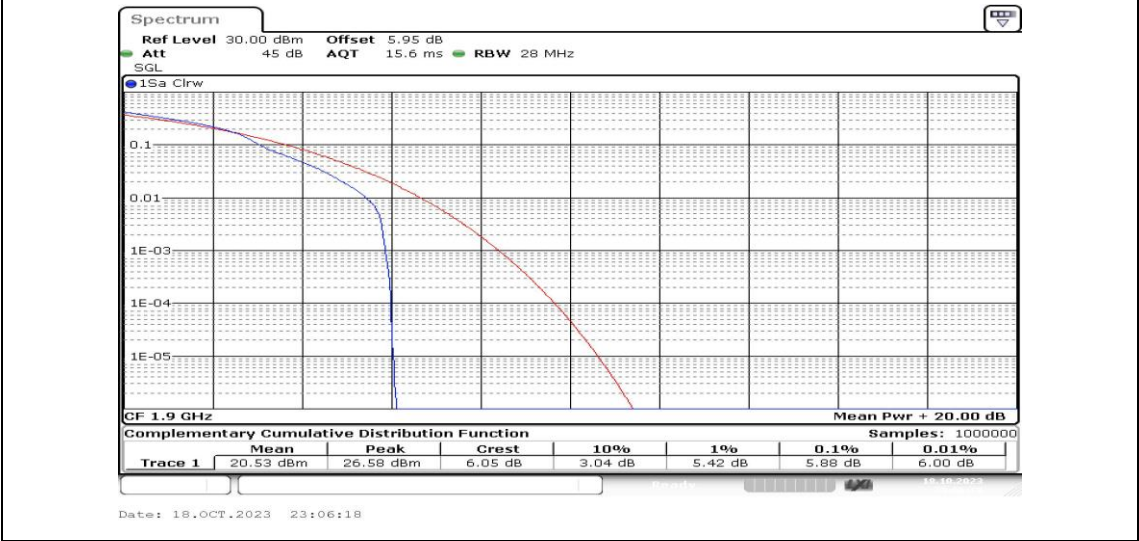
Band2-20MHz-16QAM-19100-1RB#0-PASS
