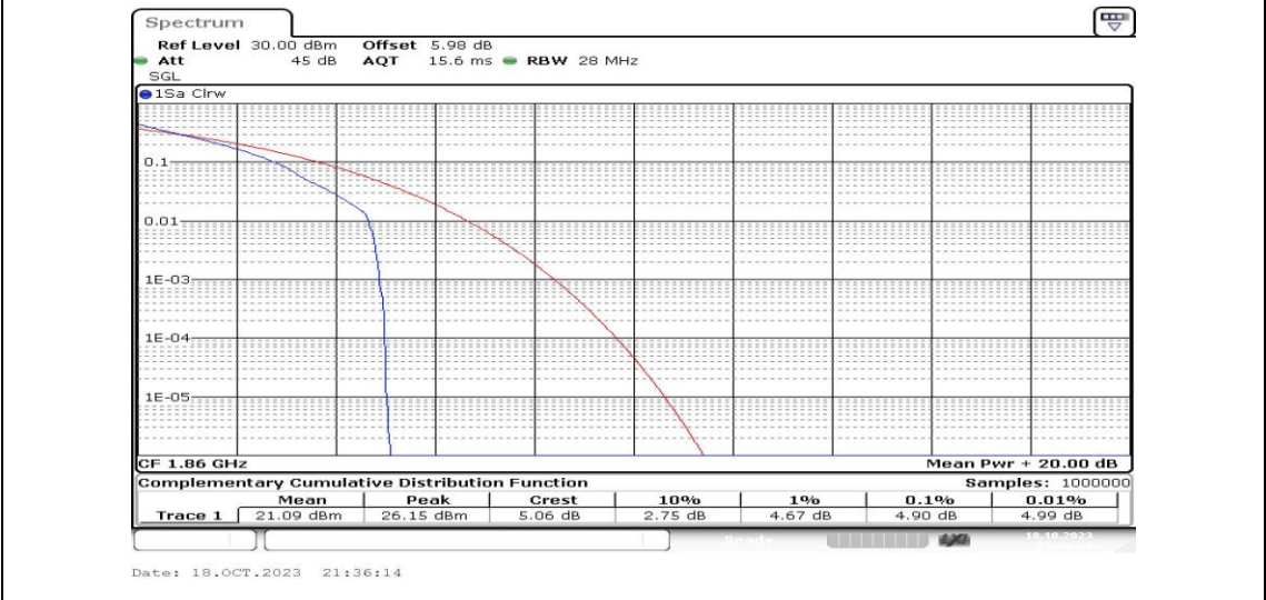
Band2-20MHz-QPSK-18700-1RB#0-PASS
