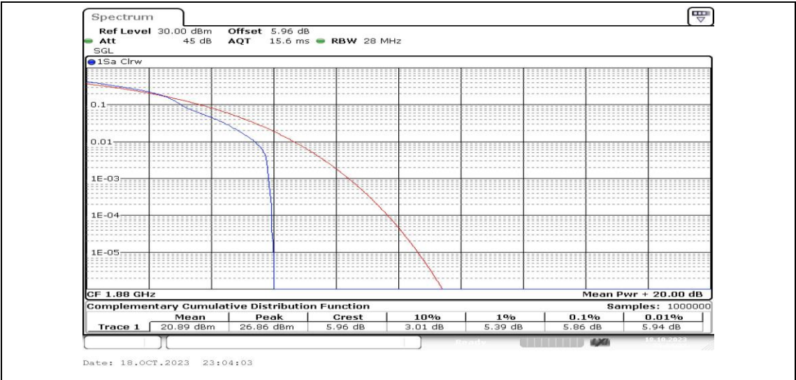
Band2-20MHz-16QAM-18900-1RB#0-PASS
