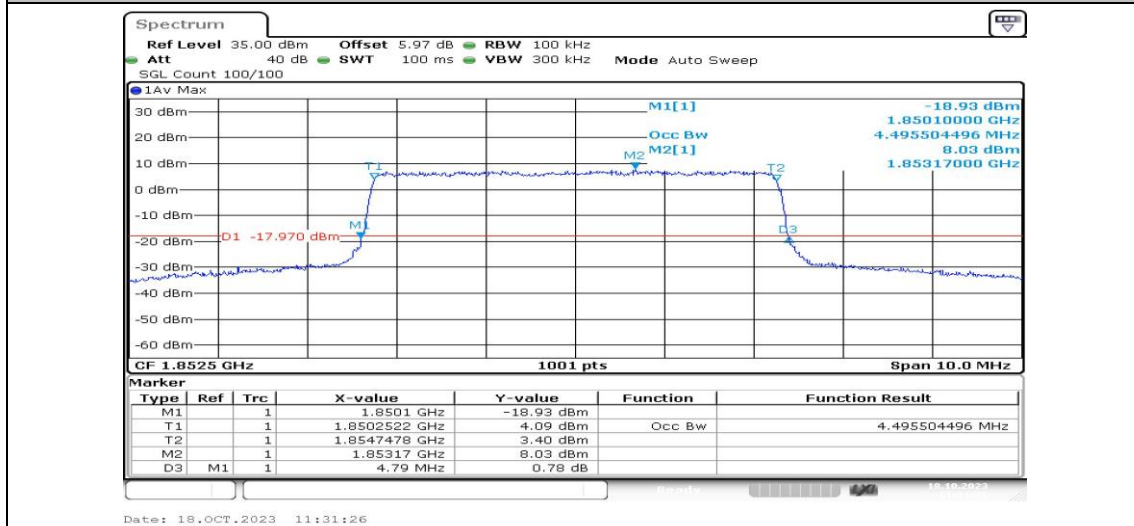
Band2-5MHz-QPSK-18625-25RB#0-PASS
