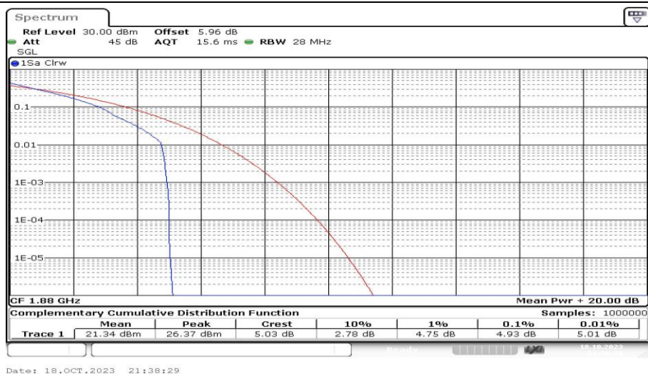
Band2-20MHz-QPSK-18900-1RB#0-PASS
