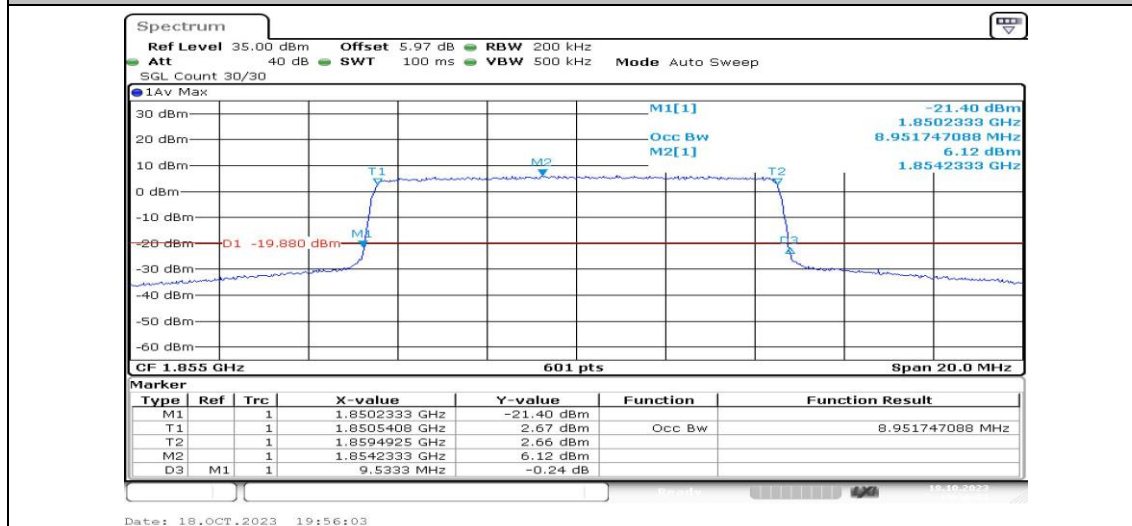
Band2-10MHz-QPSK-18650-50RB#0-PASS
