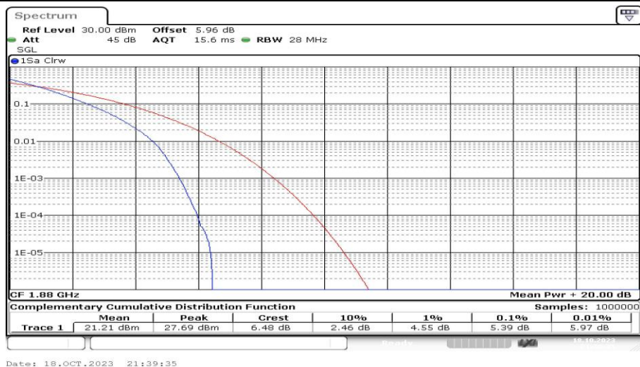
Band2-20MHz-QPSK-18900-100RB#0-PASS
