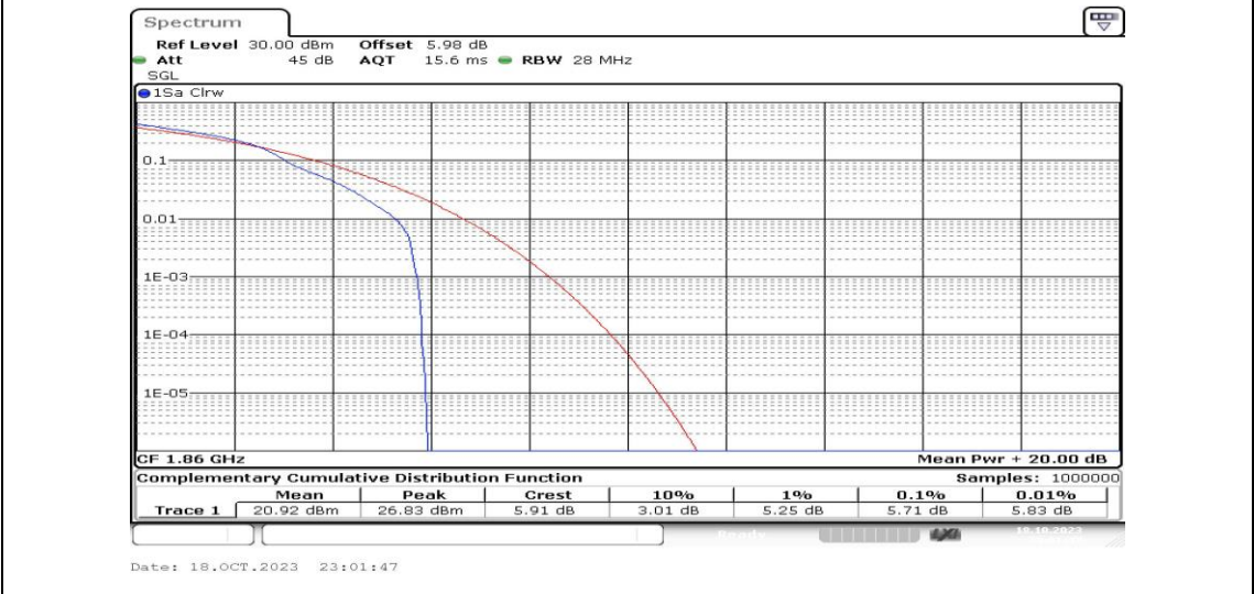
Band2-20MHz-16QAM-18700-1RB#0-PASS
