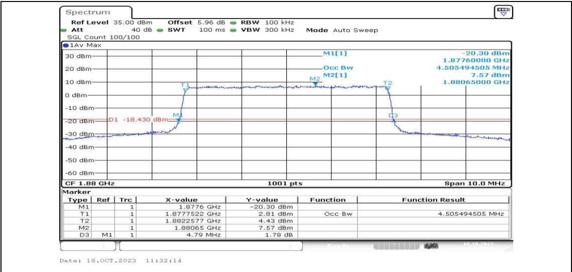
Band2-5MHz-QPSK-18900-25RB#0-PASS
