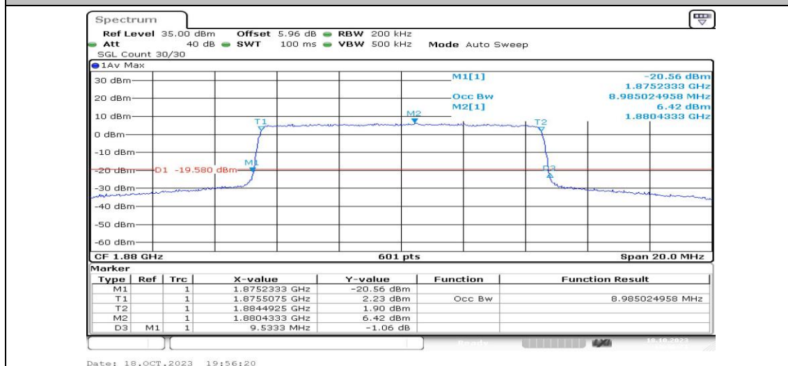
Band2-10MHz-QPSK-18900-50RB#0-PASS
