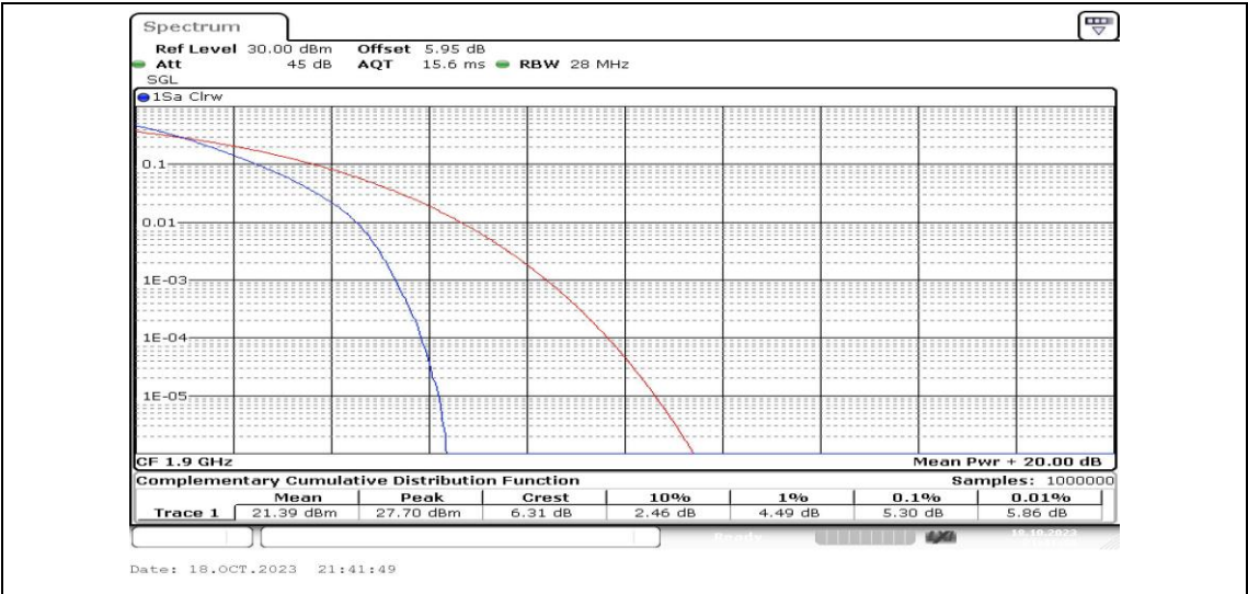
Band2-20MHz-QPSK-19100-100RB#0-PASS
