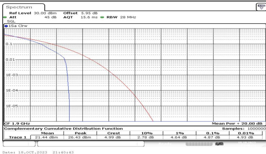
Band2-20MHz-QPSK-19100-1RB#0-PASS
