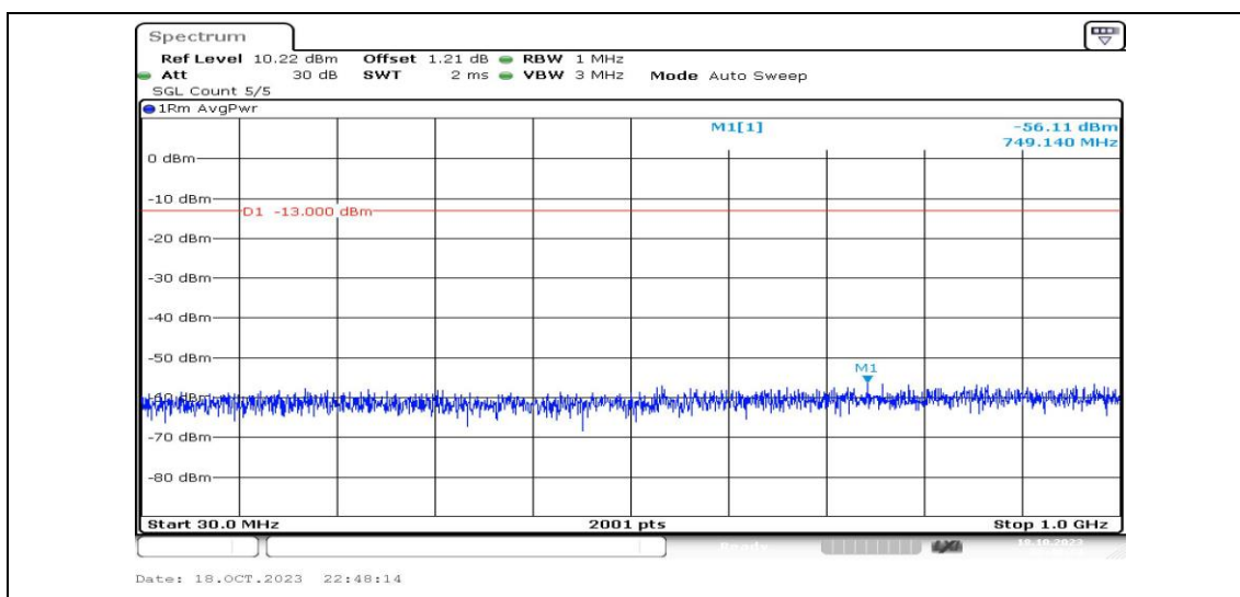
Band2-20MHz-16QAM-18700-1RB#0-Range3:30~1000MHz-PASS
