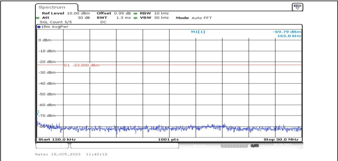
Band2-5MHz-QPSK-19175-1RB#0-Range2:0.15~30MHz-PASS
