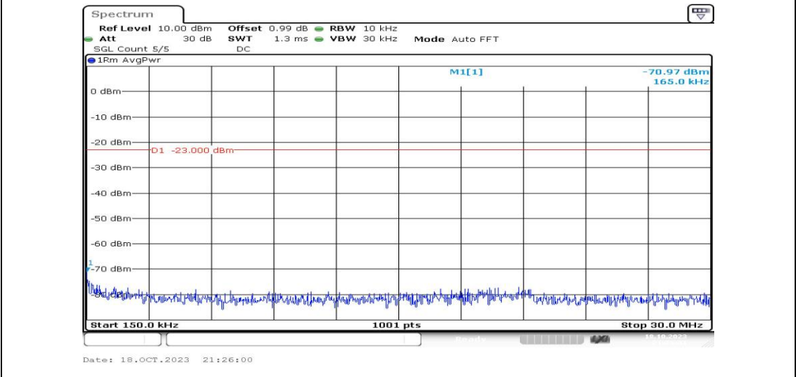
Band2-20MHz-QPSK-19100-1RB#0-Range2:0.15~30MHz-PASS
