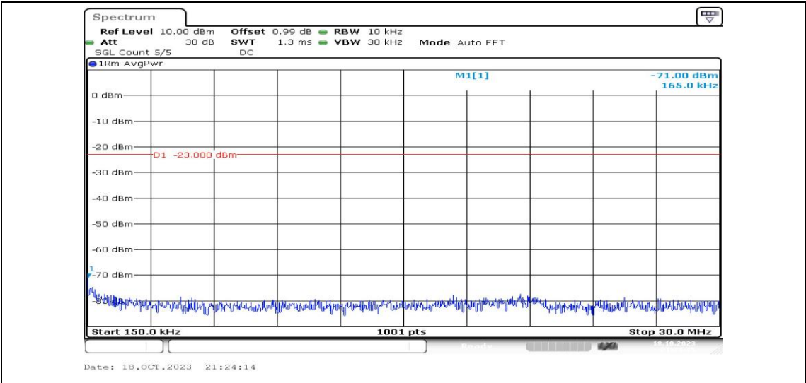
Band2-20MHz-QPSK-18900-1RB#0-Range2:0.15~30MHz-PASS
