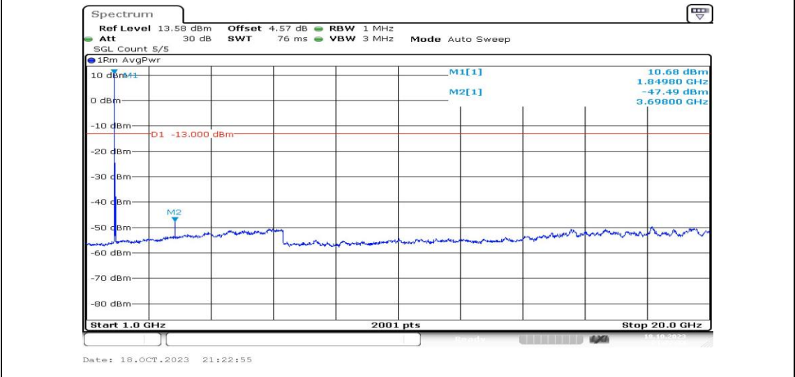
Band2-20MHz-QPSK-18700-1RB#0-Range4:1000~20000MHz-PASS
