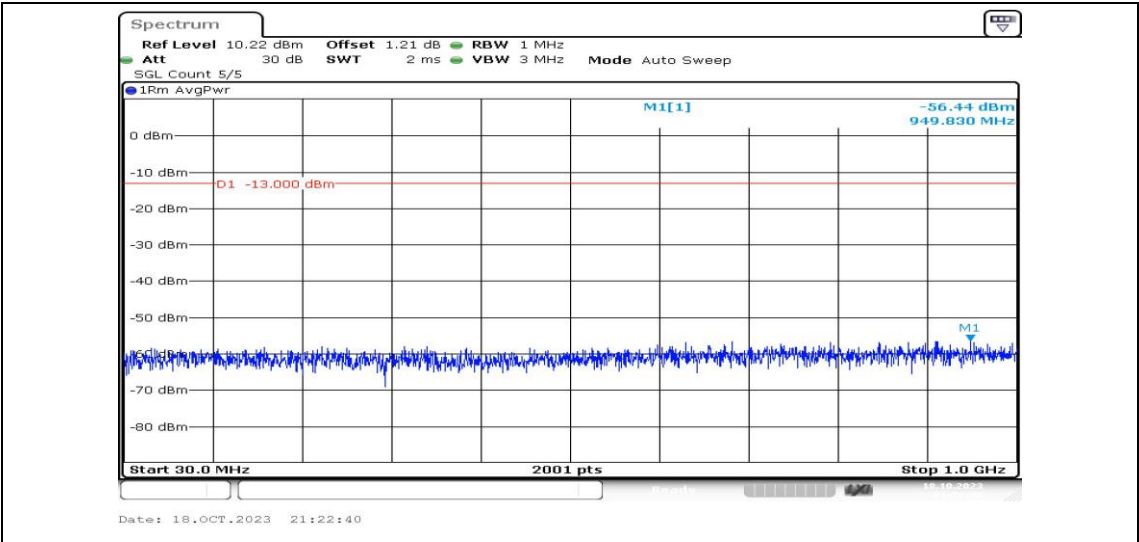
Band2-20MHz-QPSK-18700-1RB#0-Range3:30~1000MHz-PASS
