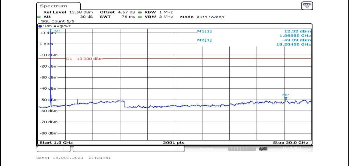
Band2-20MHz-QPSK-18900-1RB#0-Range4:1000~20000MHz-PASS
