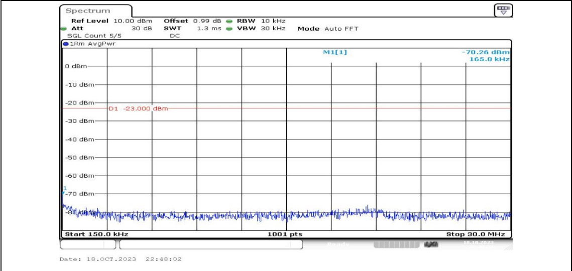
Band2-20MHz-16QAM-18700-1RB#0-Range2:0.15~30MHz-PASS
