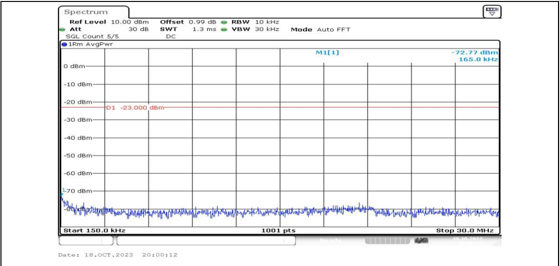
Band2-10MHz-QPSK-18900-1RB#0-Range2:0.15~30MHz-PASS
