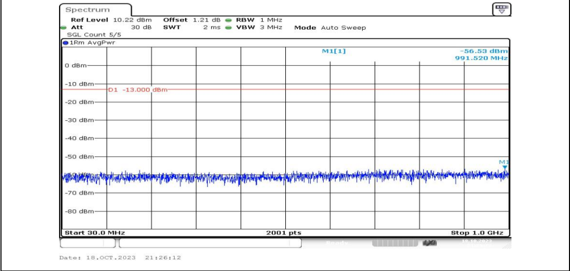
Band2-20MHz-QPSK-19100-1RB#0-Range3:30~1000MHz-PASS
