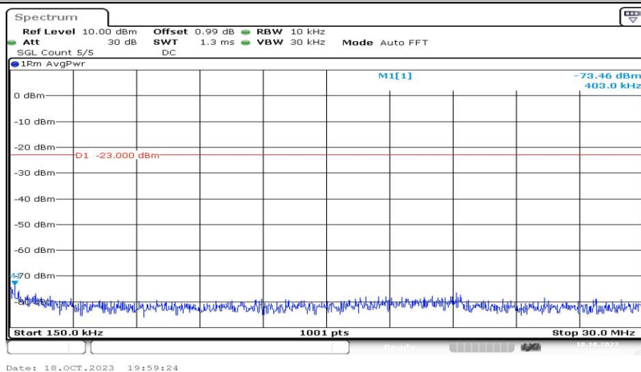
Band2-10MHz-QPSK-18650-1RB#0-Range2:0.15~30MHz-PASS
