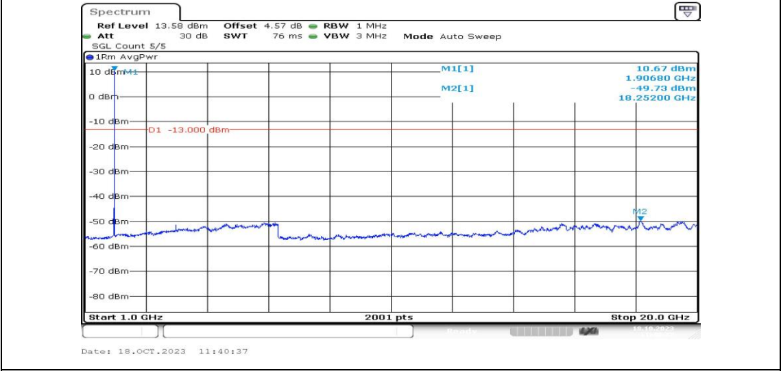
Band2-5MHz-QPSK-19175-1RB#0-Range4:1000~20000MHz-PASS
