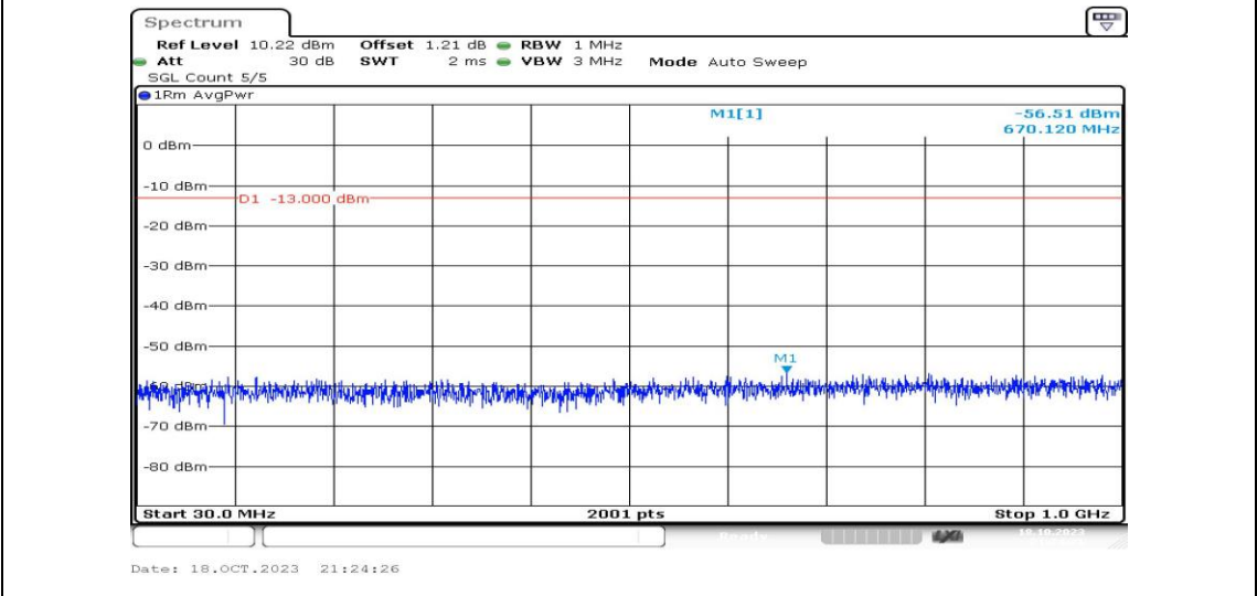
Band2-20MHz-QPSK-18900-1RB#0-Range3:30~1000MHz-PASS
