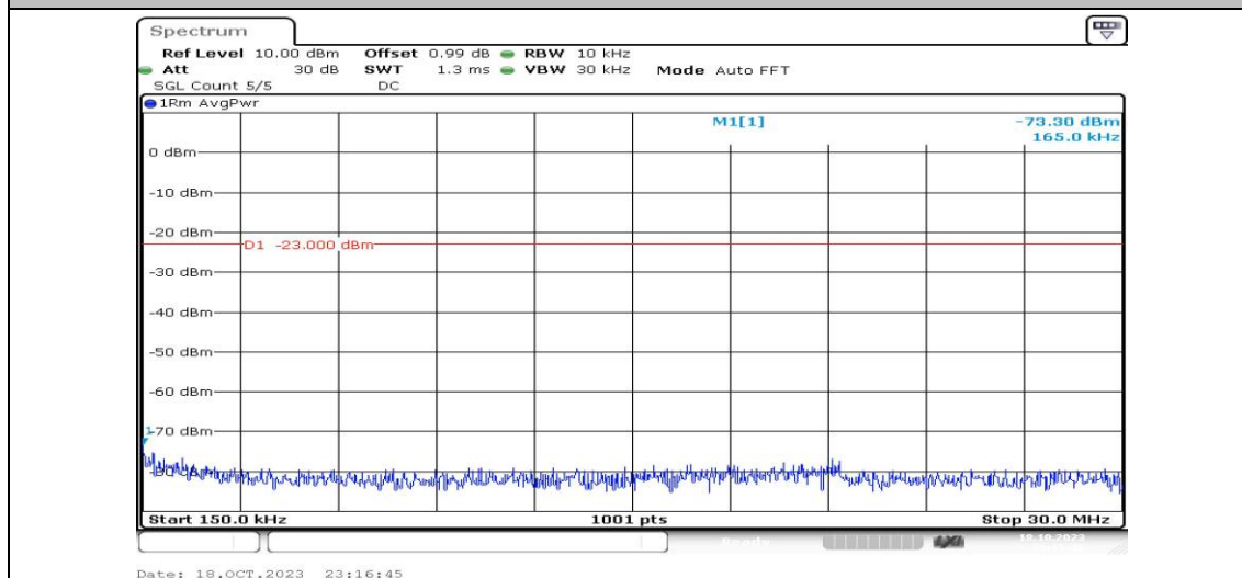
Band4-10MHz-QPSK-20000-1RB#0-Range2:0.15~30MHz-PASS
