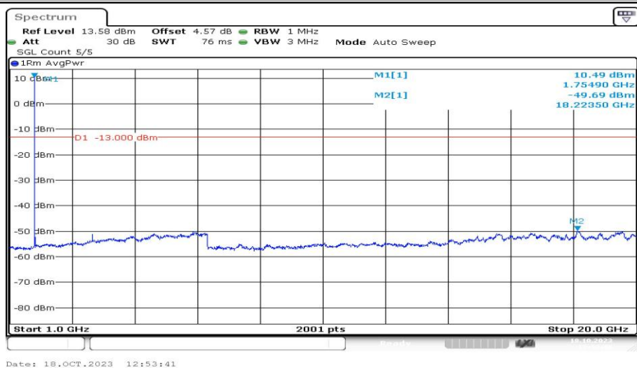
Band4-5MHz-QPSK-20375-1RB#0-Range4:1000~20000MHz-PASS
