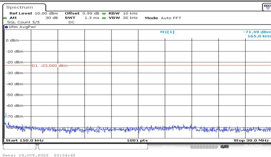
Band4-15MHz-QPSK-20025-1RB#0-Range2:0.15~30MHz-PASS
