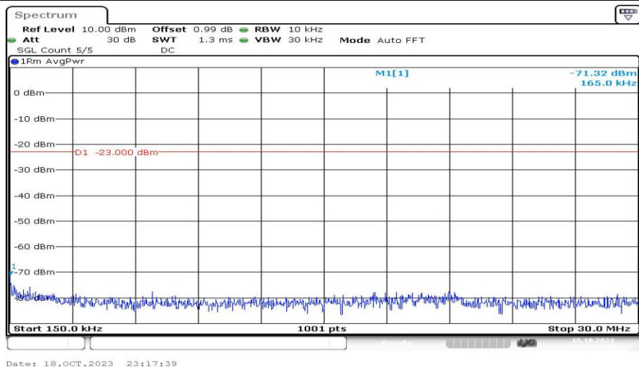
Band4-10MHz-QPSK-20175-1RB#0-Range2:0.15~30MHz-PASS
