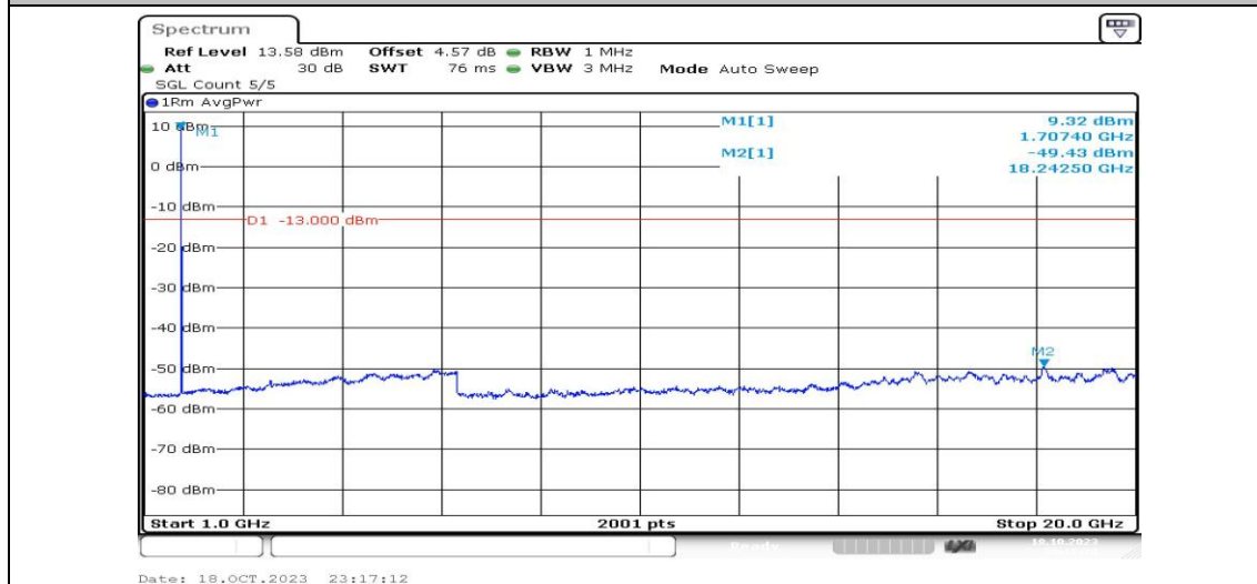
Band4-10MHz-QPSK-20000-1RB#0-Range4:1000~20000MHz-PASS
