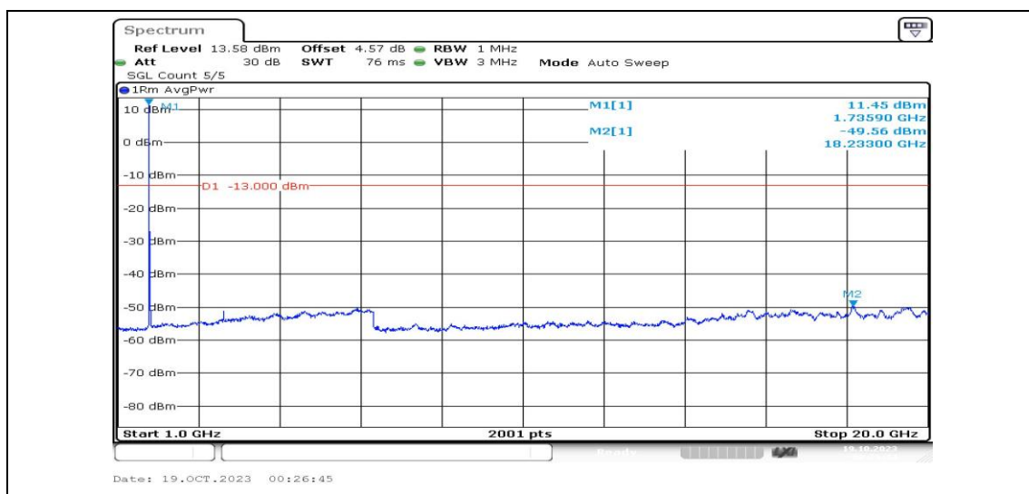
Band4-20MHz-QPSK-20300-1RB#0-Range4:1000~20000MHz-PASS
