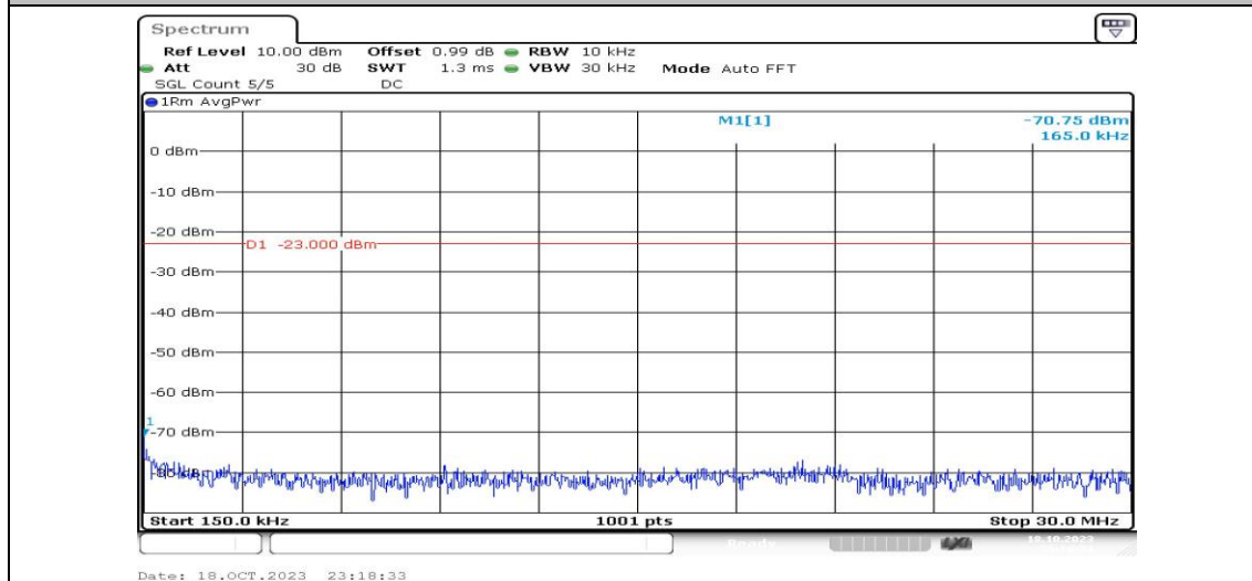
Band4-10MHz-QPSK-20350-1RB#0-Range2:0.15~30MHz-PASS
