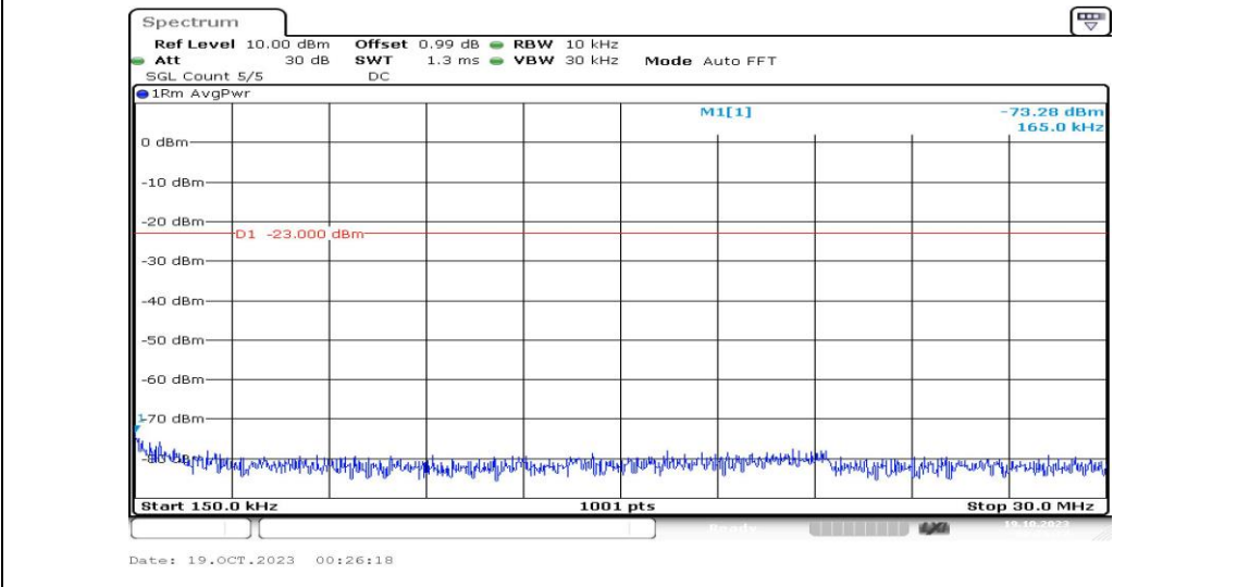
Band4-20MHz-QPSK-20300-1RB#0-Range2:0.15~30MHz-PASS
