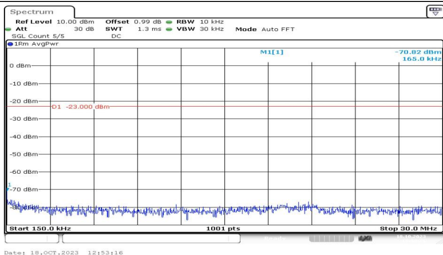
Band4-5MHz-QPSK-20375-1RB#0-Range2:0.15~30MHz-PASS
