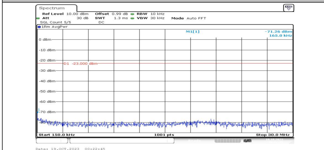
Band4-20MHz-QPSK-20050-1RB#0-Range2:0.15~30MHz-PASS
