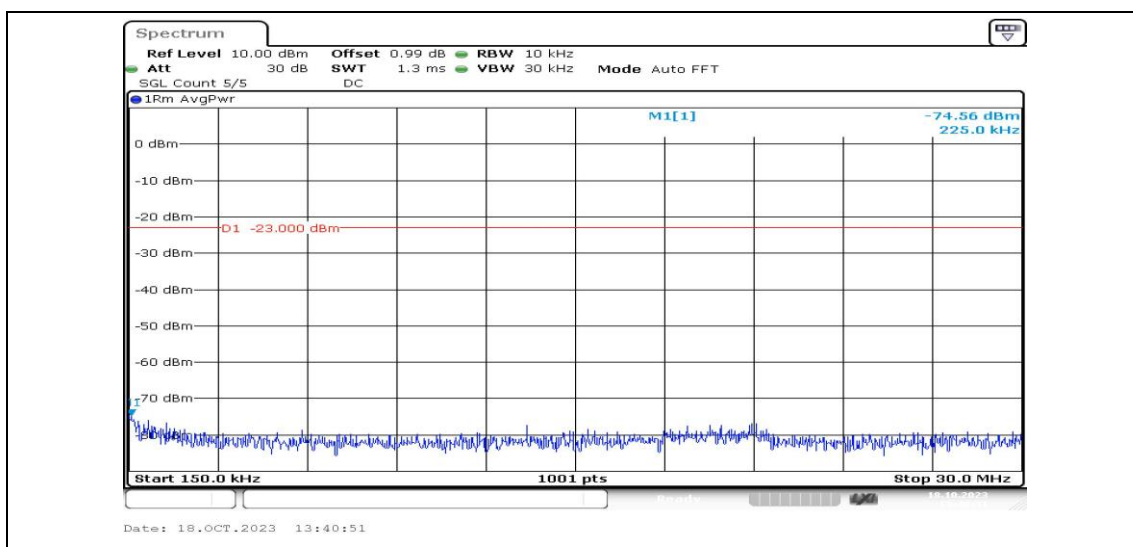
Band5-3MHz-QPSK-20635-1RB#0-Range2:0.15~30MHz-PASS
