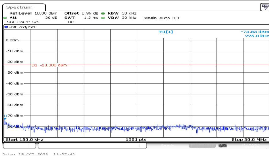
Band5-3MHz-QPSK-20415-1RB#0-Range2:0.15~30MHz-PASS
