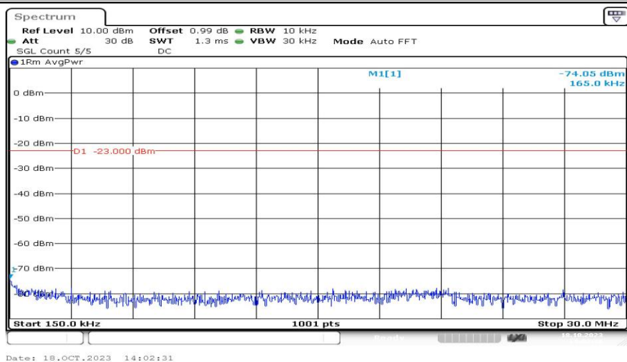
Band5-5MHz-QPSK-20425-1RB#0-Range2:0.15~30MHz-PASS
