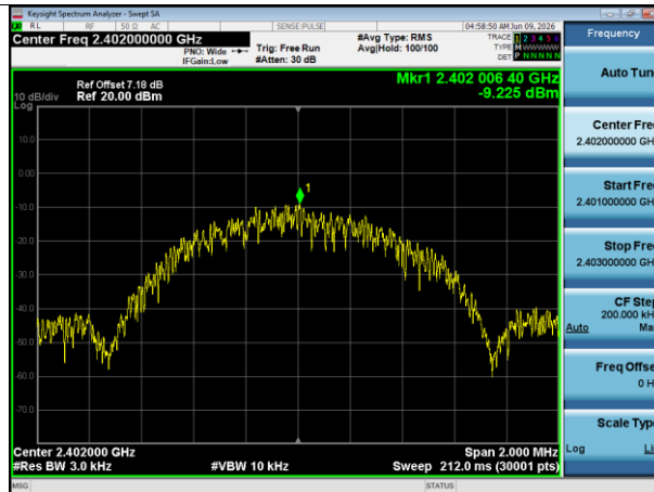
PSD NVNT BLE 1M 2402MHz Ant1
