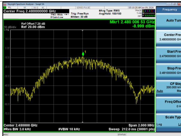
PSD NVNT BLE 1M 2480MHz Ant1
