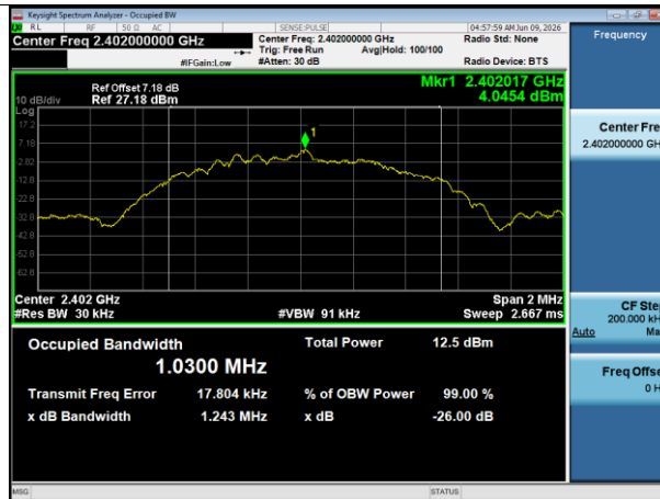
OBW NVNT BLE 1M 2402MHz Ant1
