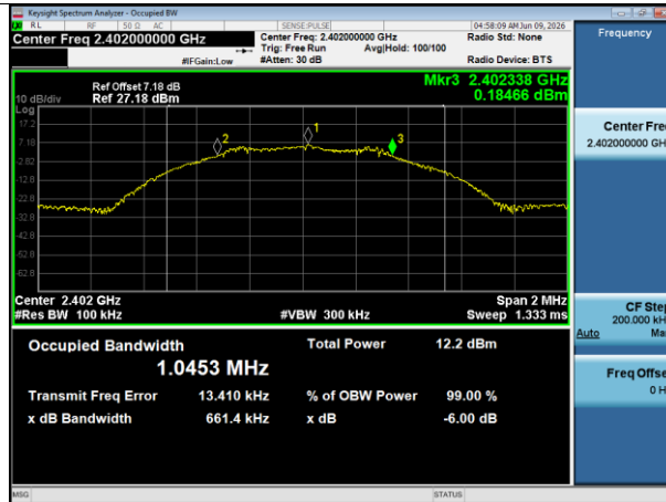
-6dB Bandwidth NVNT BLE 1M 2402MHz Ant1
