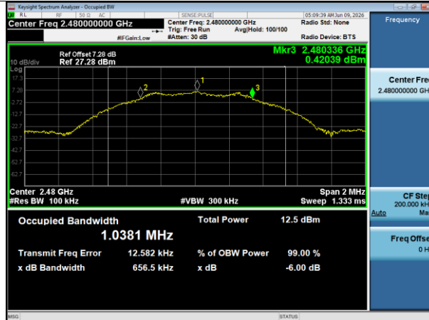
-6dB Bandwidth NVNT BLE 1M 2480MHz Ant1
