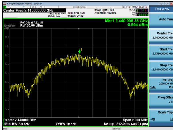
PSD NVNT BLE 1M 2440MHz Ant1
