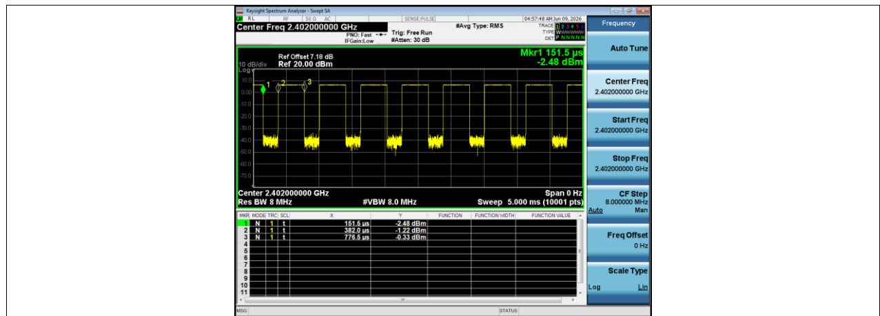
Duty Cycle NVNT BLE 1M 2402MHz Ant1
