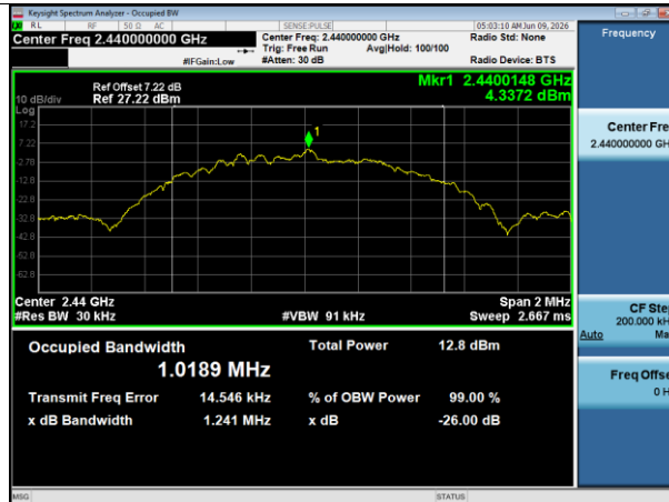
OBW NVNT BLE 1M 2440MHz Ant1
