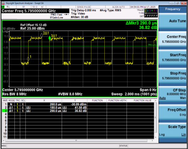
NTNV-11AC40MIMO-Ant1-5795
