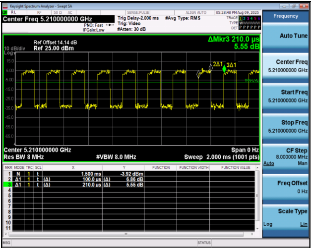
NTNV-11AC80MIMO-Ant1-5210
