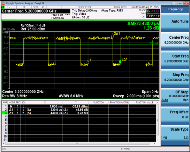
NTNV-11AX20MIMO-Ant2-5200
