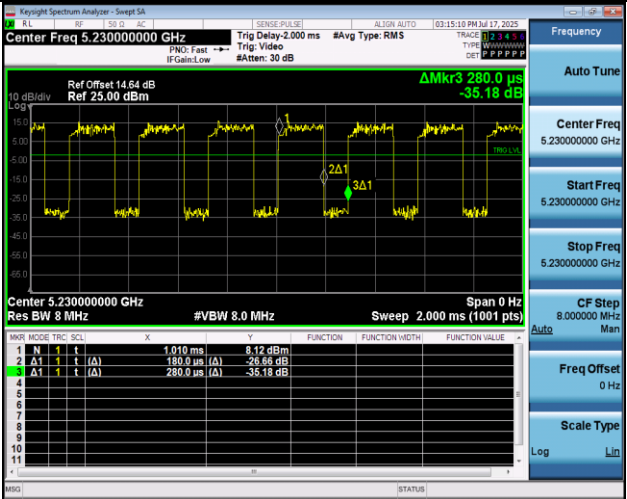
NTNV-11AC40MIMO-Ant1-5230
