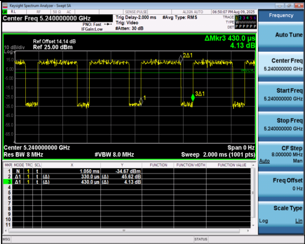
NTNV-11AX20MIMO-Ant1-5240
