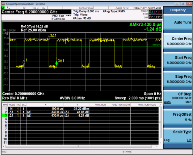
NTNV-11AX20MIMO-Ant1-5200
