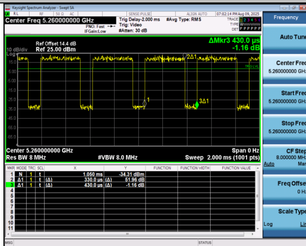
NTNV-11AX20MIMO-Ant1-5260
