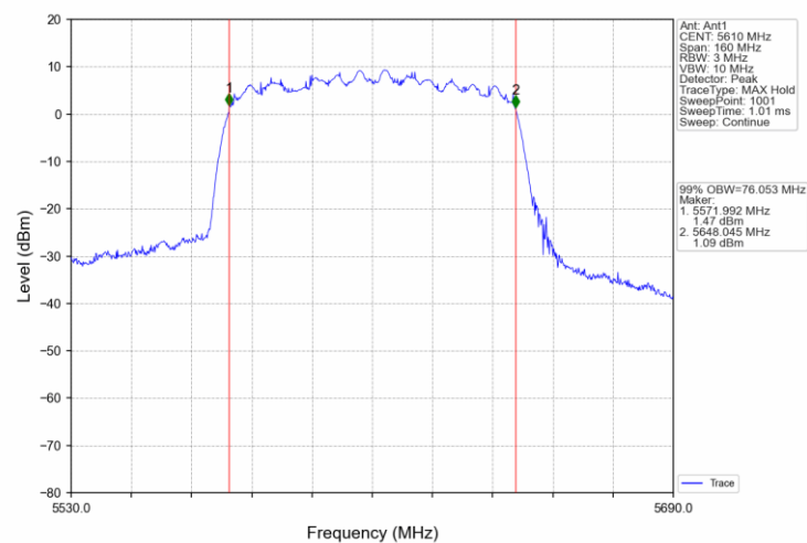
802.11ac(VHT80)_HCH_5690MHz_AntB_NTNV
