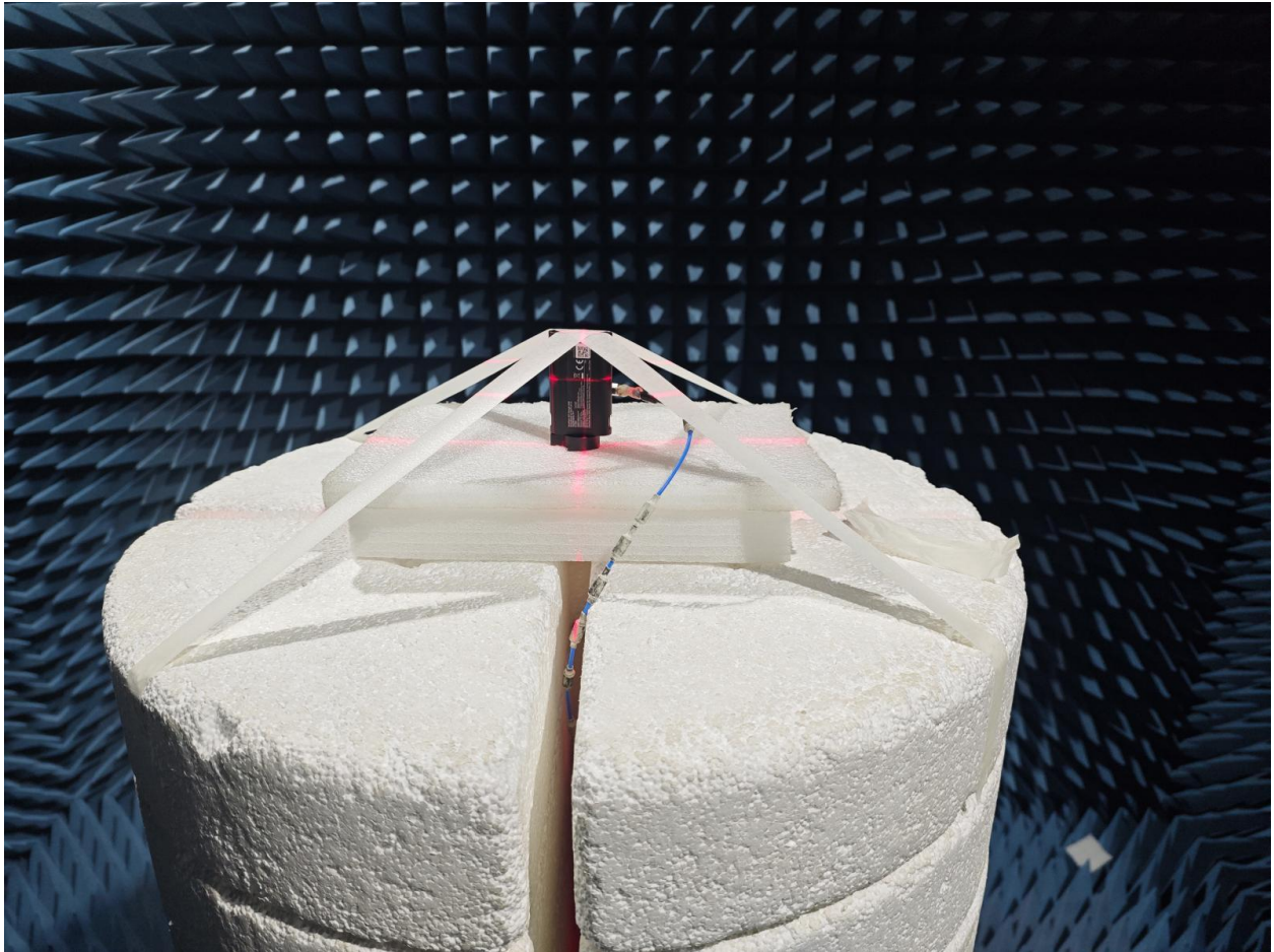
DUT Setup Photo
