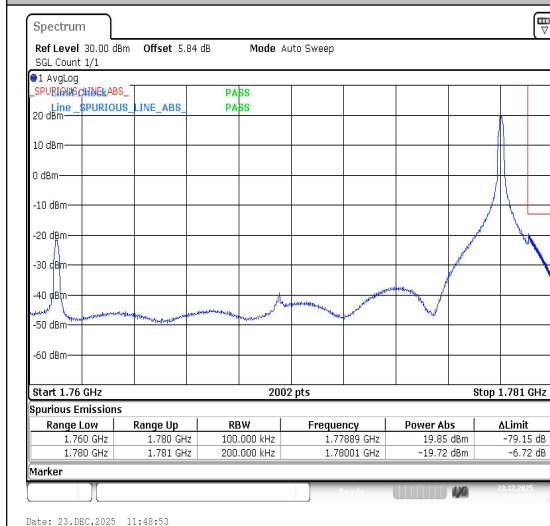
Band66-20MHz-QPSK-132572-1RB#99-PASS
