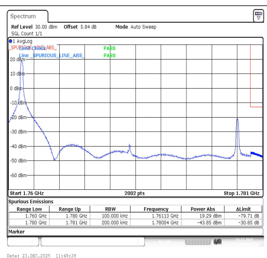
Band66-20MHz-QPSK-132572-1RB#0-PASS
