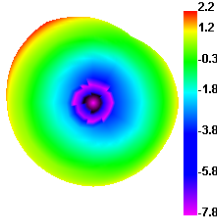
2450.000MHz
