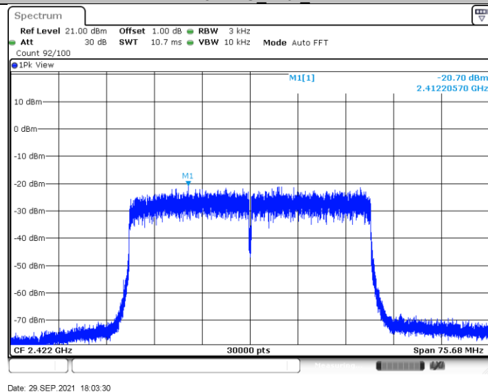
11AX40MIMO_Ant1_2422
