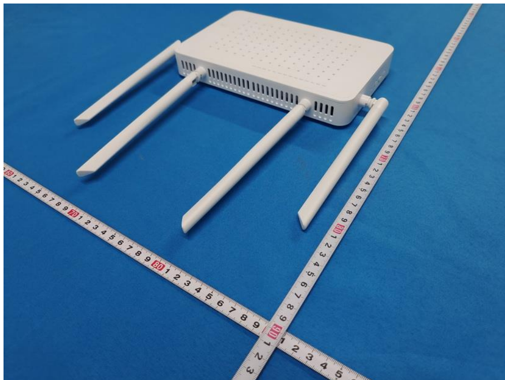
Model: TA1910-4GVC-W
