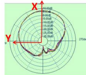
E2 (Phi=90)
