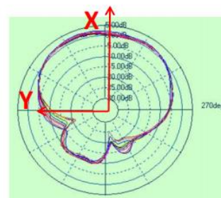
E2 ( Phi=90 )
