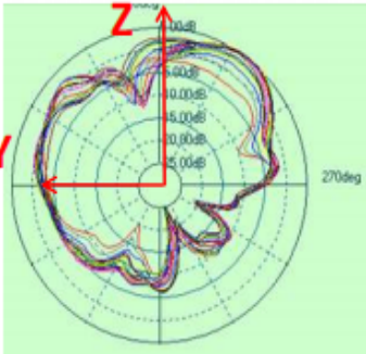
E1 (Phi=0)
