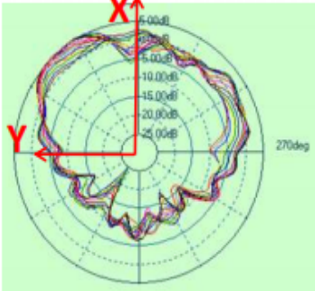
E2 (Phi=90)
