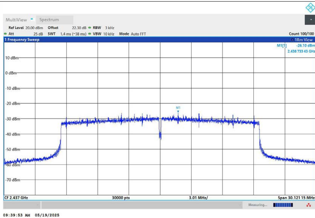
11AX20MIMO-Ant1-2437-PASS
