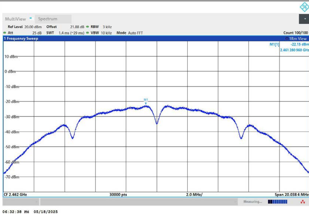
11B-Ant2-2462-PASS
