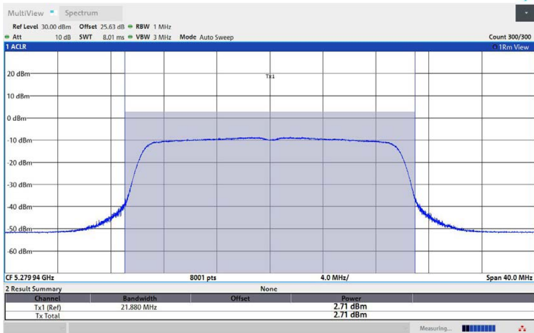
11AX20MIMO-Ant1-5280-TPC_H-PASS
