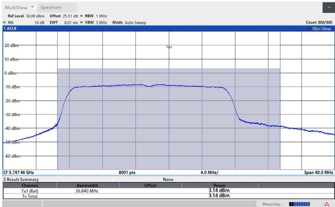
11AX20MIMO-Ant3-5745-PASS
