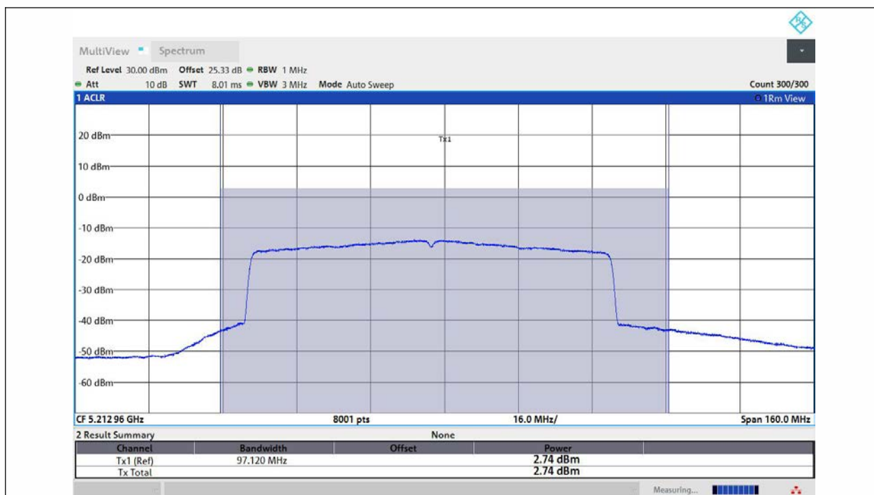
11AX80MIMO-Ant1-5210-PASS
