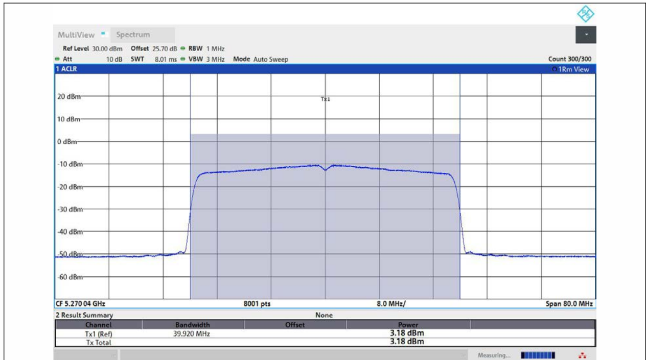
11AX40MIMO-Ant1-5270-TPC_H-PASS
