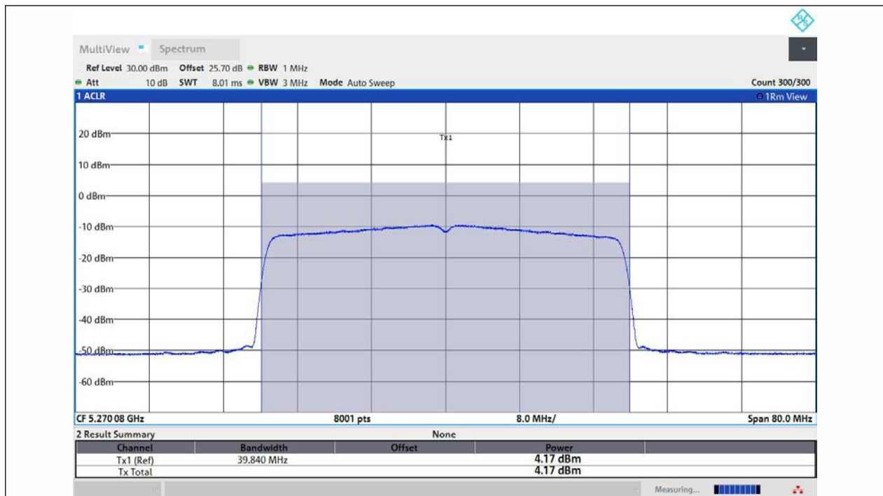
11AX40MIMO-Ant3-5270-TPC_H-PASS
