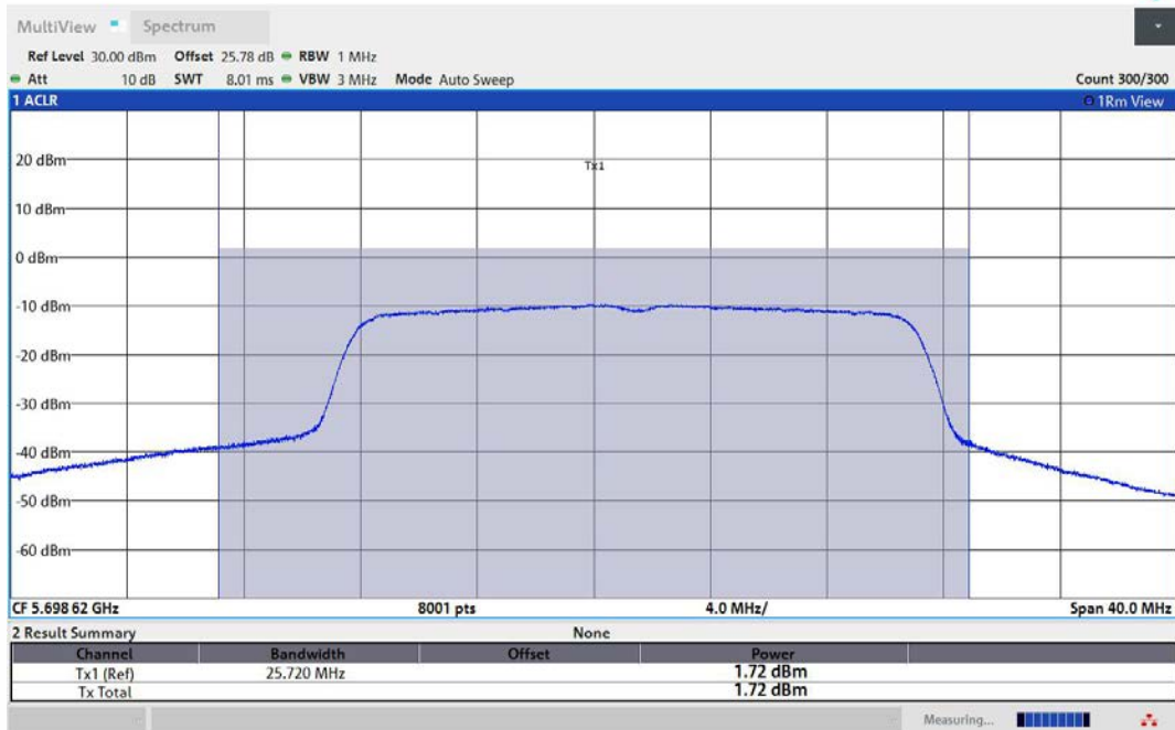
11AX20MIMO-Ant1-5700-TPC_H-PASS
