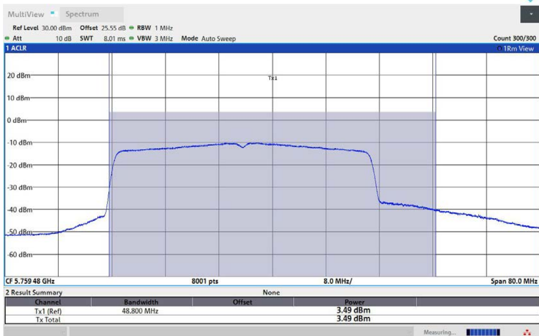
11AX40MIMO-Ant3-5755-PASS
