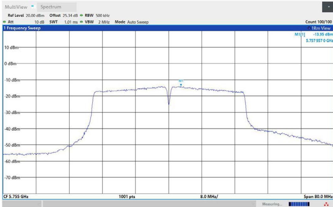
11N40MIMO-Ant1-5755-PASS
