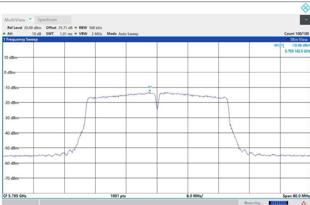
11N40MIMO-Ant1-5795-PASS
