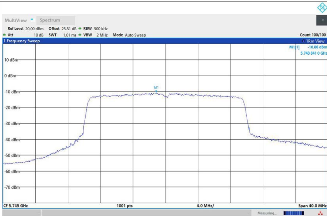
11AX20MIMO-Ant3-5745-PASS
