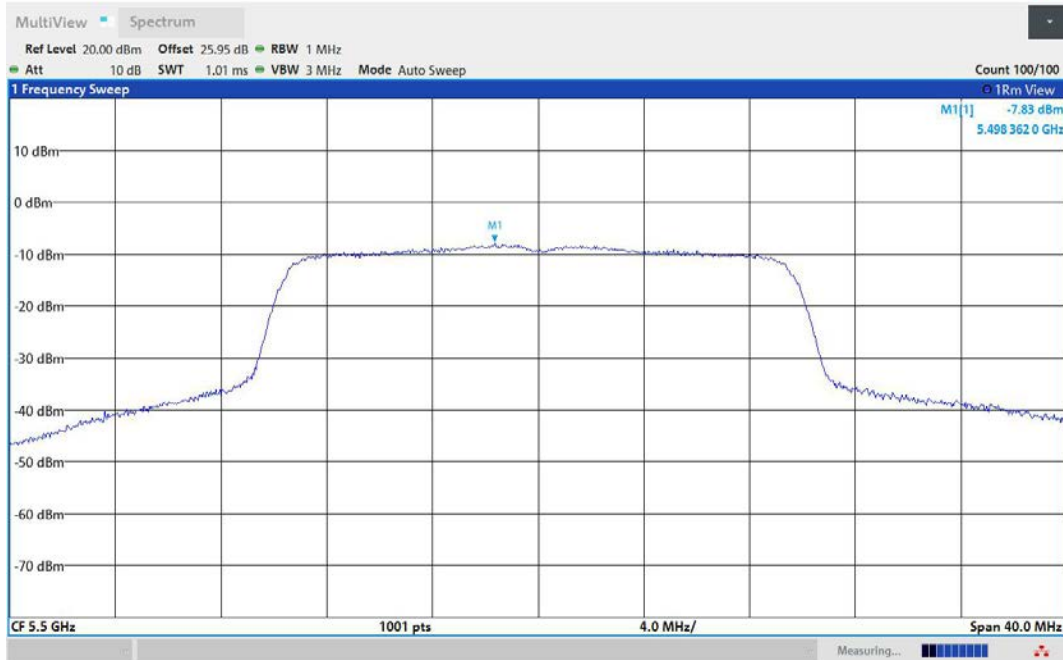
11AX20MIMO-Ant1-5500-PASS
