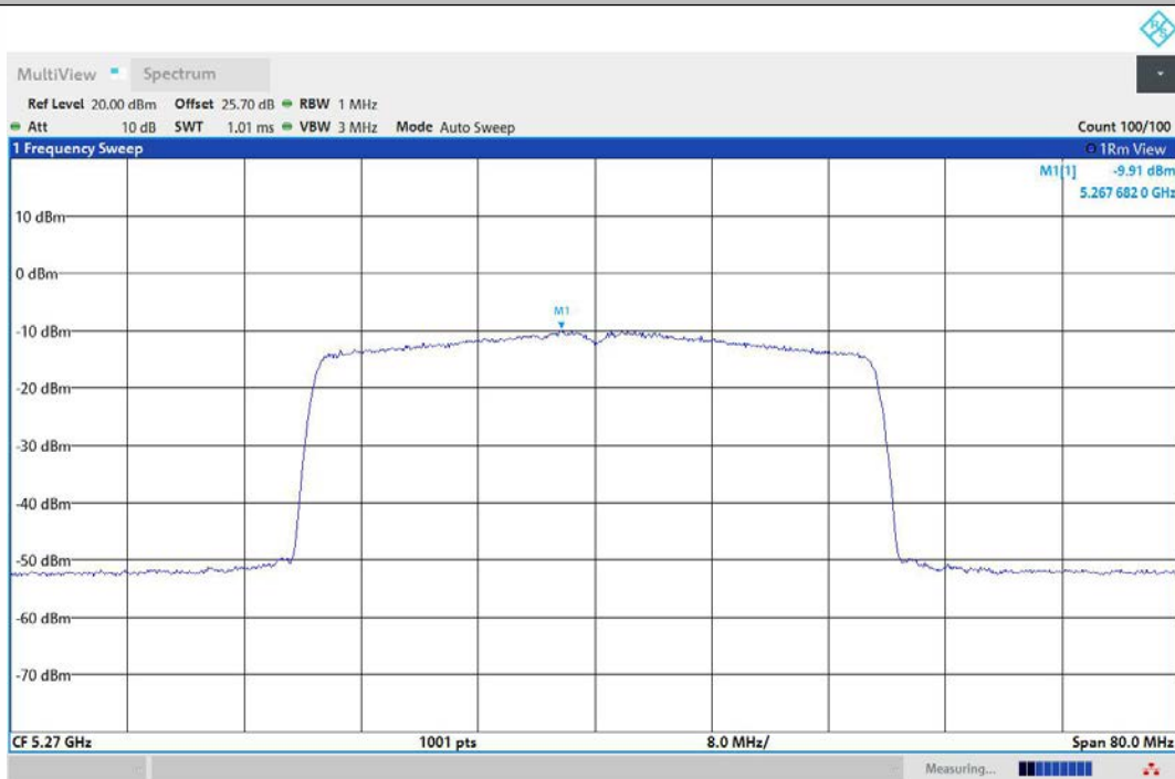
11AX40MIMO-Ant1-5270-PASS
