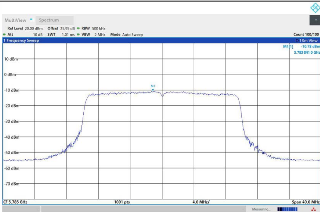
11AX20MIMO-Ant1-5785-PASS
