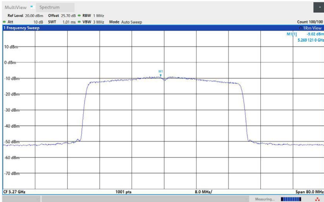
11AX40MIMO-Ant3-5270-PASS
