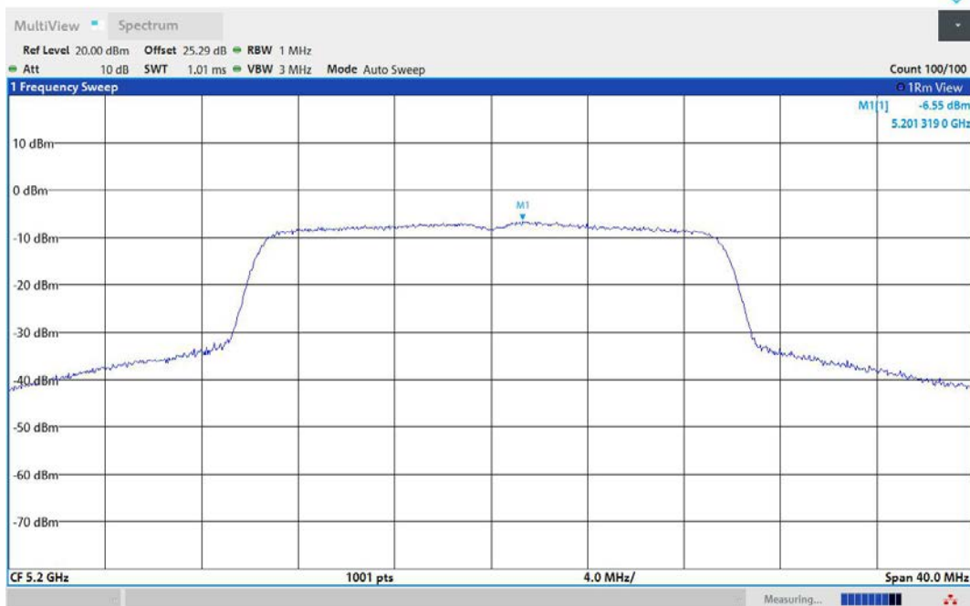
11AX20MIMO-Ant3-5200-PASS
