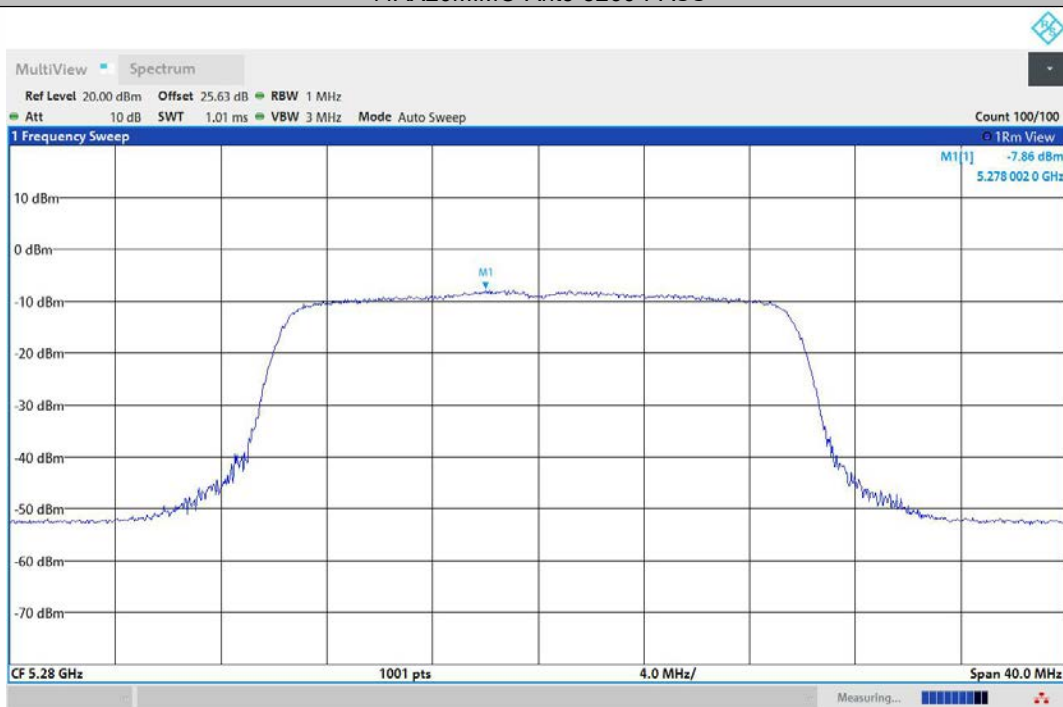
11AX20MIMO-Ant1-5280-PASS
