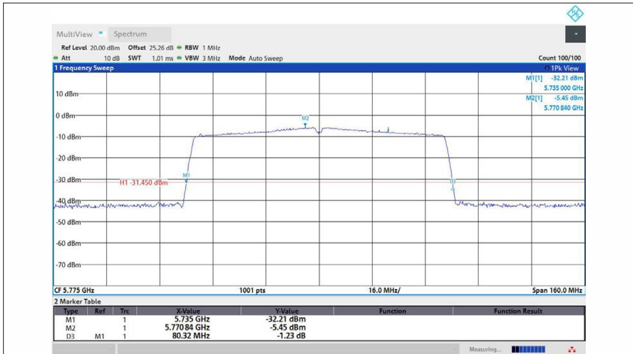
11AC80MIMO-Ant1-5775
