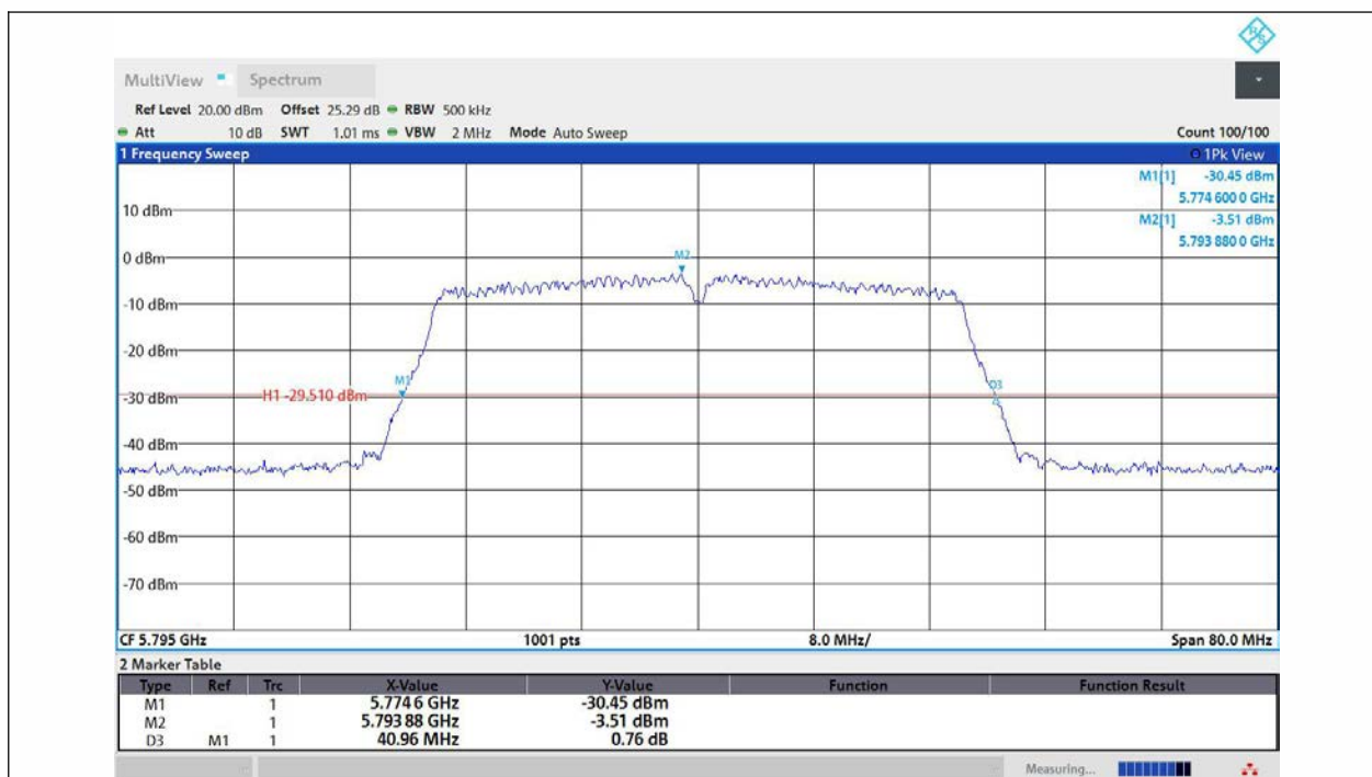
11N40MIMO-Ant3-5795
