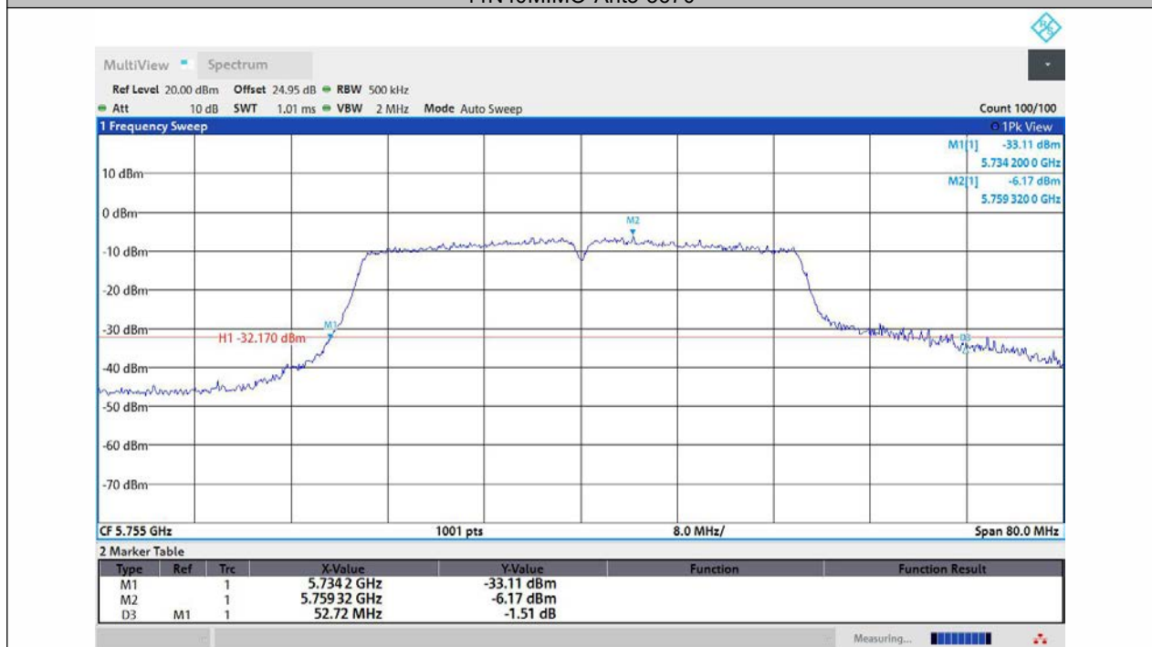
11N40MIMO-Ant1-5755
