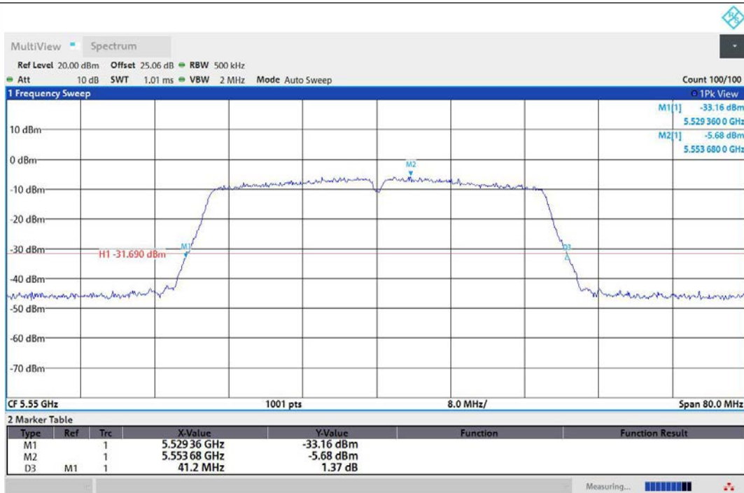
11AC40MIMO-Ant1-5550
