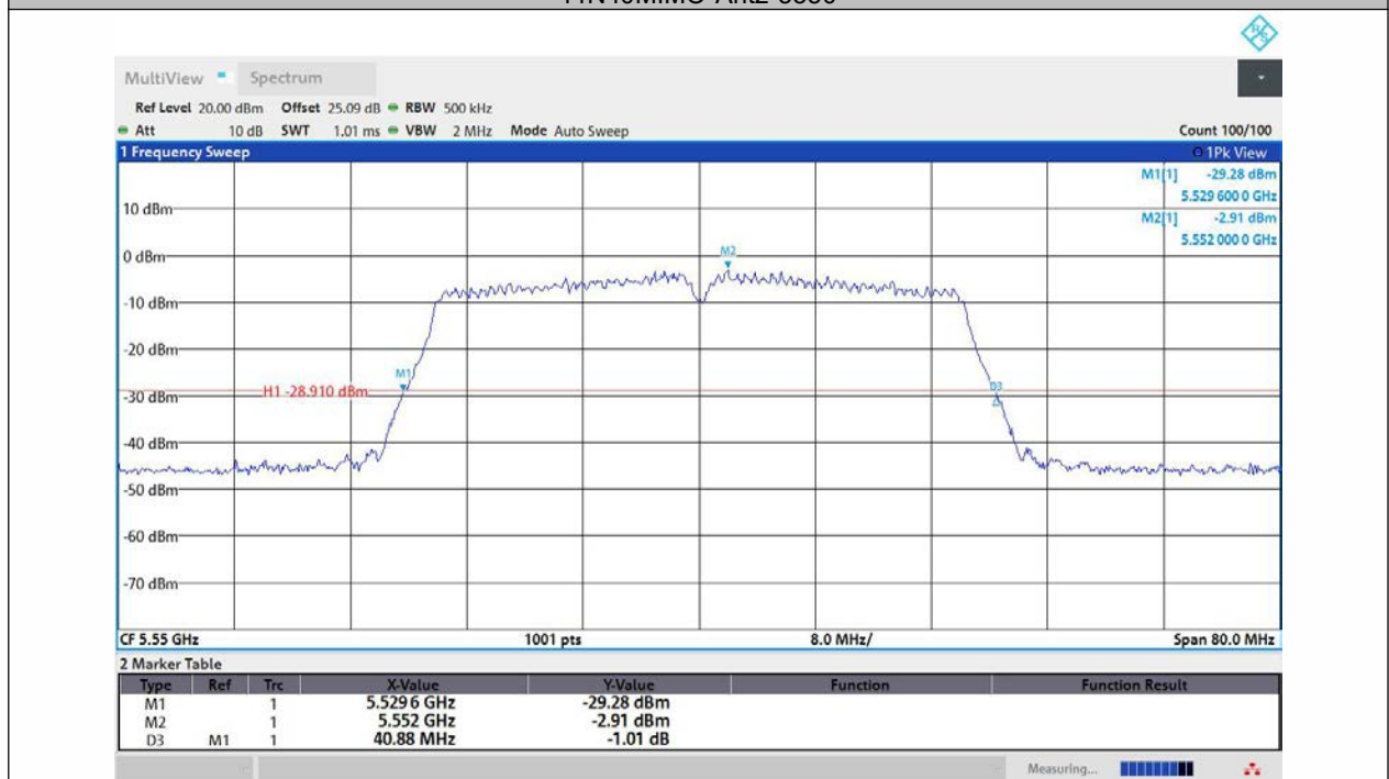
11N40MIMO-Ant3-5550
