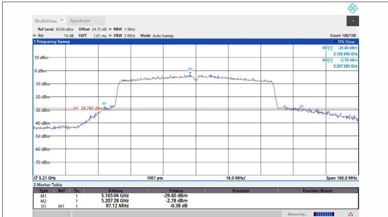
11AC80MIMO-Ant3-5210
